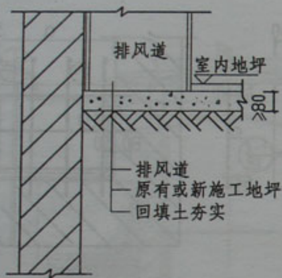
原有或新施工地坪上安装排风道
