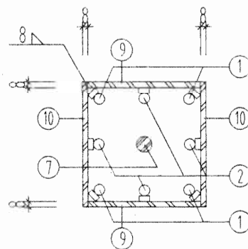
A-A 剖面
