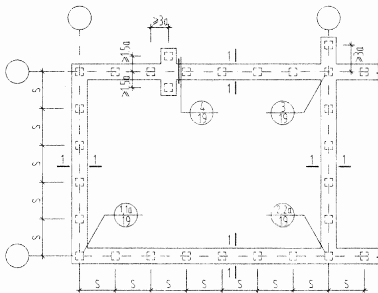
桩基础平面示意图
