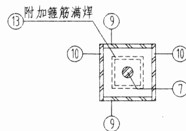
B-B剖面
