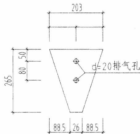
⑨ 钢板详图 \delta = 8
