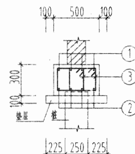
1-1(用于A型)
