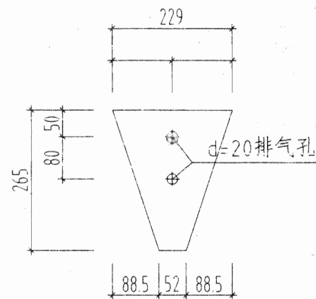
⑩ 钢板详图 \delta = 8
