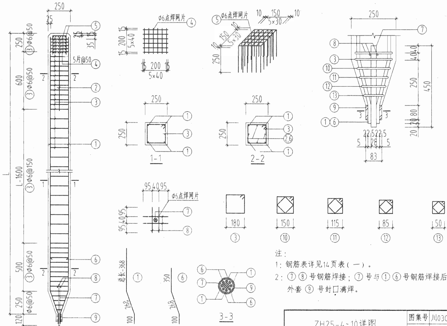
ZH25-4~10详图
