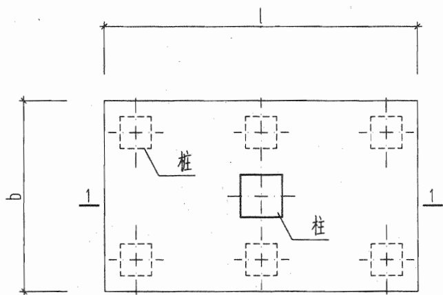
桩基础平面示意图
