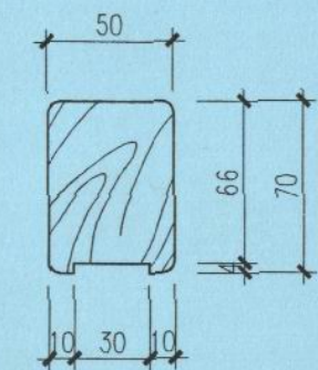
木扶手断面
