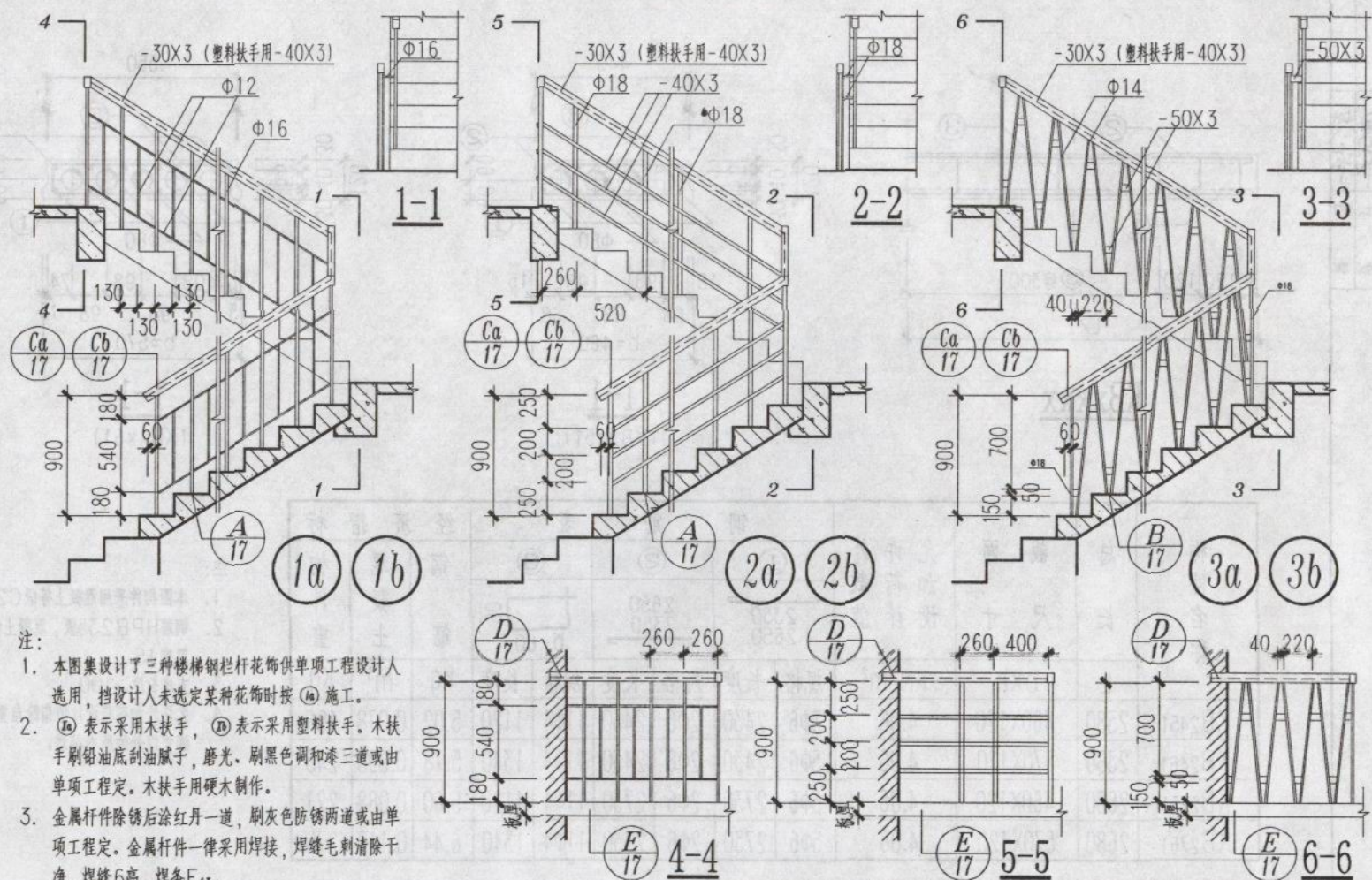
楼梯钢栏杆
