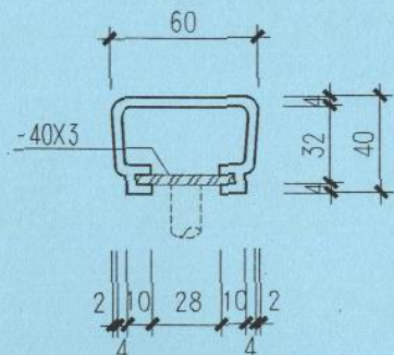
塑料扶手断面
