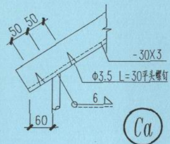
木扶手断面
