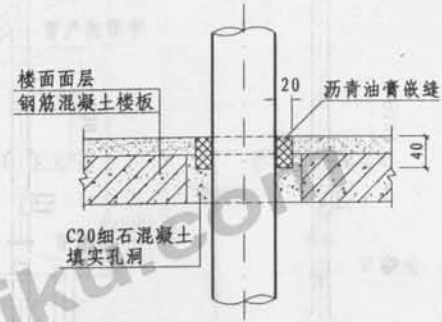
穿楼面 (III型)
