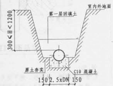
混凝土基础
