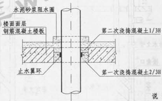
穿楼面 (V型)
