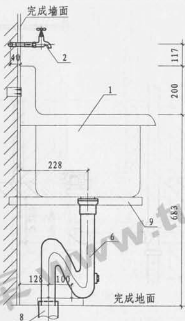
污水盆側面
