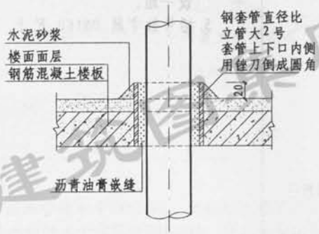
穿楼面 (IV型)
