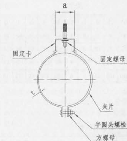
立剖面 (横管)
