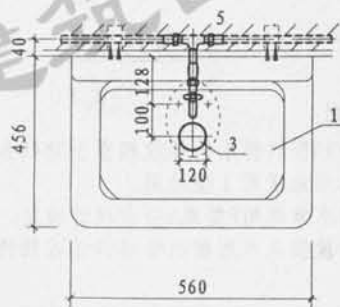
污水盆平面
