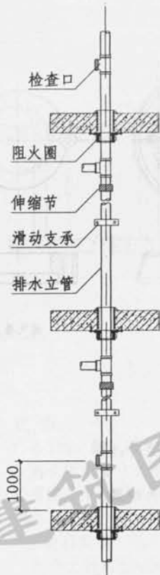
单立管
