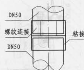
转换接头 II
