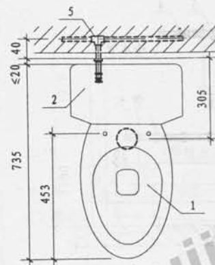
平面图
