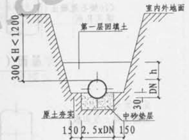
砂垫层基础
