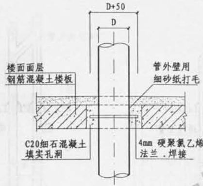
穿楼面 (II型)
