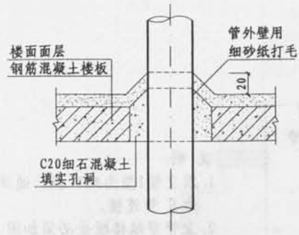
穿楼面 (I 型)
