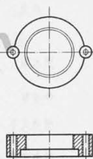
通气盖座
