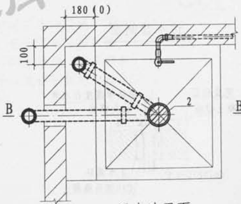
污水池平面
