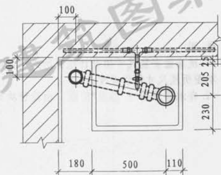
洗涤盆平面
