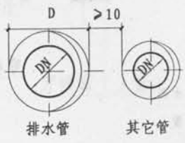
楼板留洞
