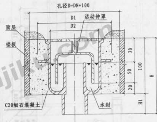
I 型地漏
