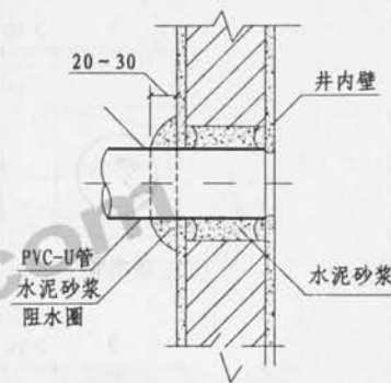
穿检查井壁
