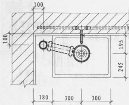
化验盆平面
