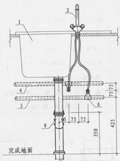
1-1剖面图
