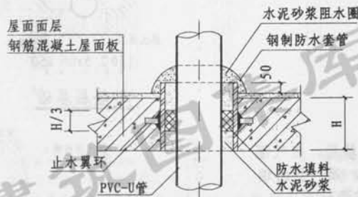
穿屋面 (III 型)
