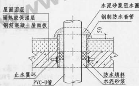
穿屋面 (IV 型)
