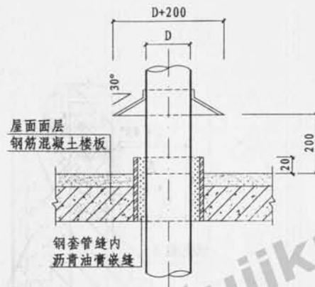
穿屋面 (II 型)
