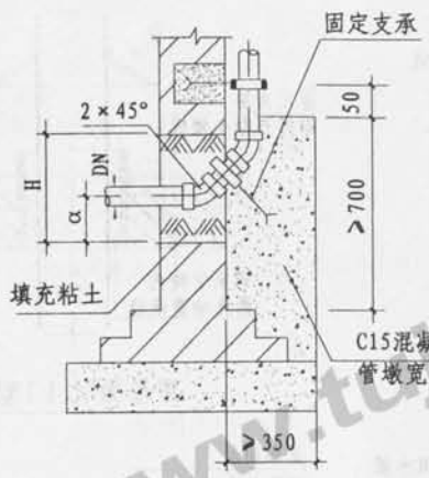
墙基留洞
