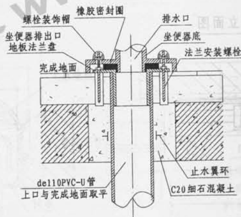
坐便器排出口详图 (法兰镶接)
