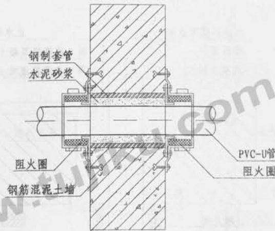
双面安装
