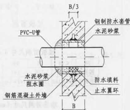
穿地下室外墙
