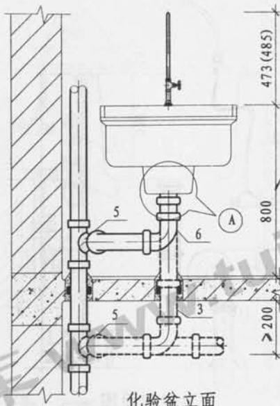
化验盆立面
