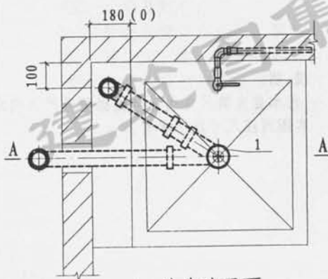
洗涤池平面
