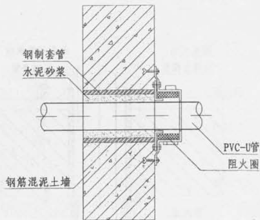
单面安装
