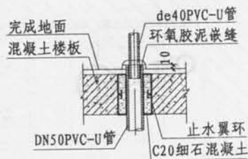
节点"C"
