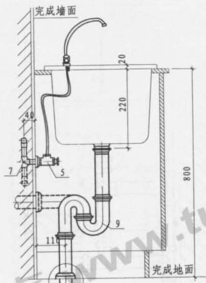
2-2剖面图
