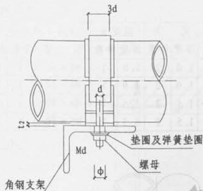
側面
