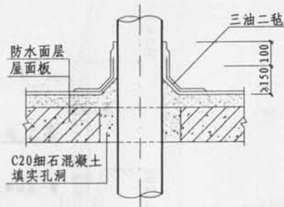
穿屋面 (I 型)
