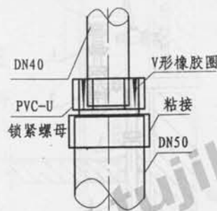
转换接头 I
