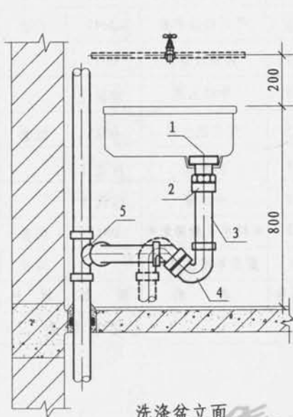
洗涤盆立面
