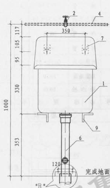
污水盆立面
