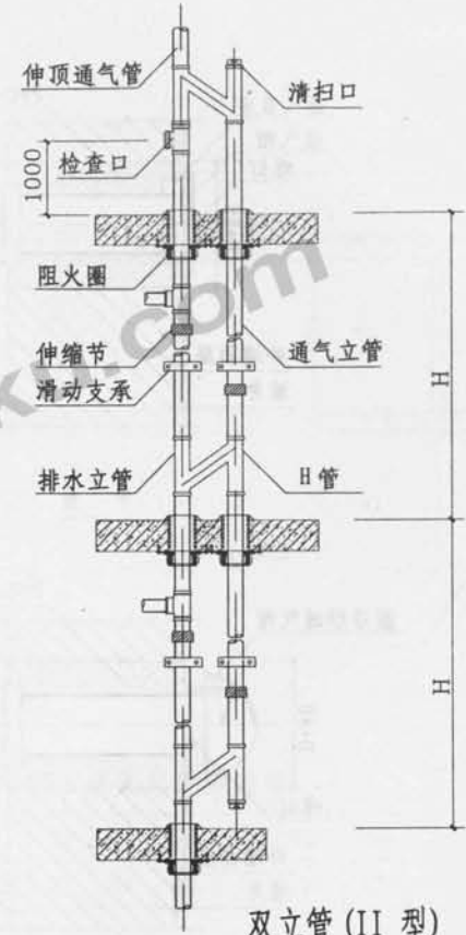
双立管 (I 型)
