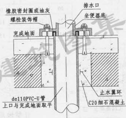
坐便器排出口详图 (无法兰镶接)
