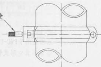
侧面 (立管)
