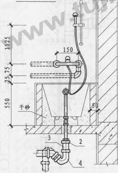
2-2剖面
