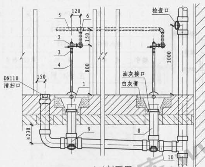
1-1剖面图
