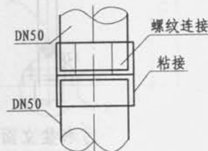
转换接头
