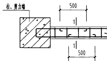
水平系梁详图
