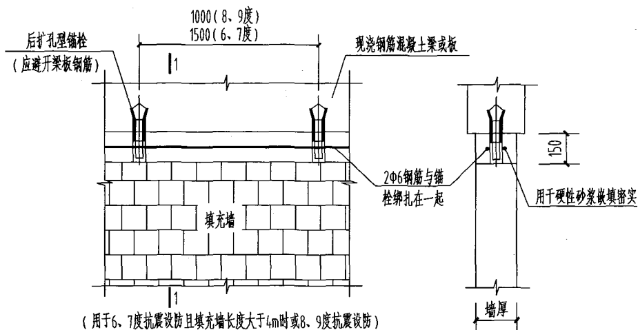
③ (墙体顶部锚栓设置大样)
