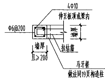
构造柱 (用于 B \geq 2\text{m} )
