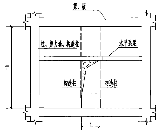
④ (用于 B \geq 2\text{m} 且 H_n > 4\text{m} )
