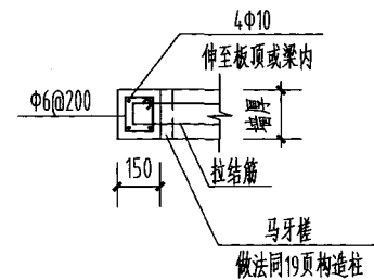
构造柱 (用于 0.6\text{m} < B < 2\text{m} )
