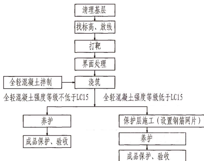
图6.2.1 全轻混凝土建筑地面保温工程施工流程图
