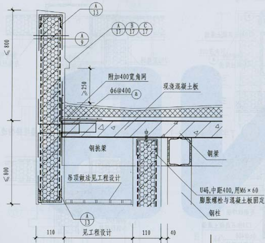
1 挑檐墙构造
