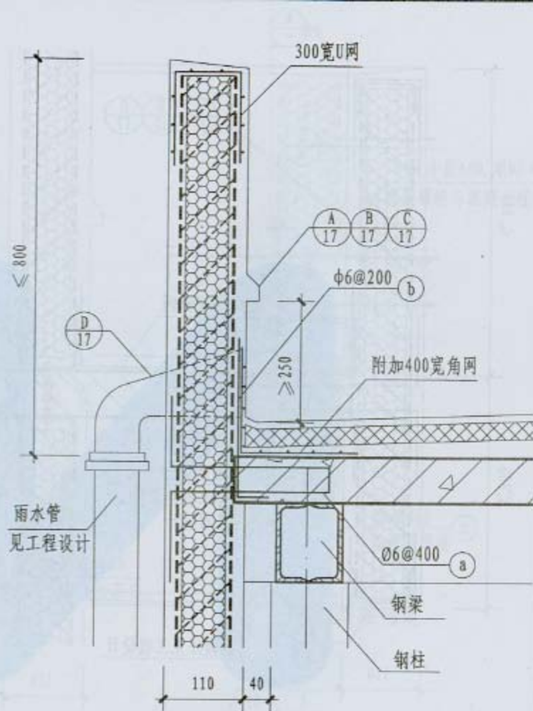
2 女儿墙连接构造(钢筋混凝土屋面)
