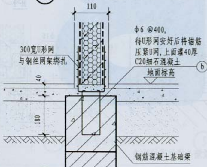
2 板墙与基础连接构造(二)
