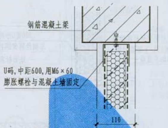
① 板墙与混凝土梁连接构造(一)
