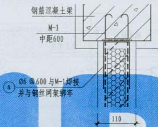
② 板墙与混凝土梁连接构造(二)
