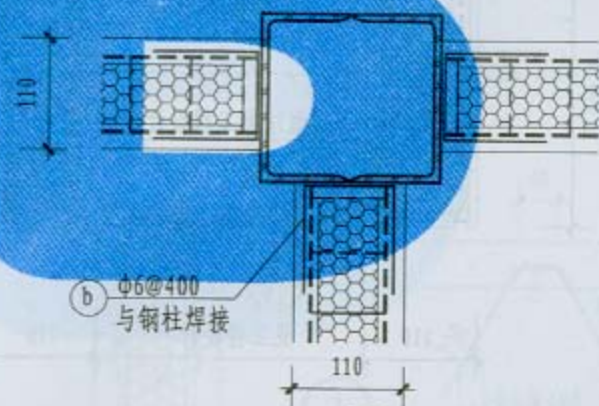
④ 丁字墙连接构造(四)
