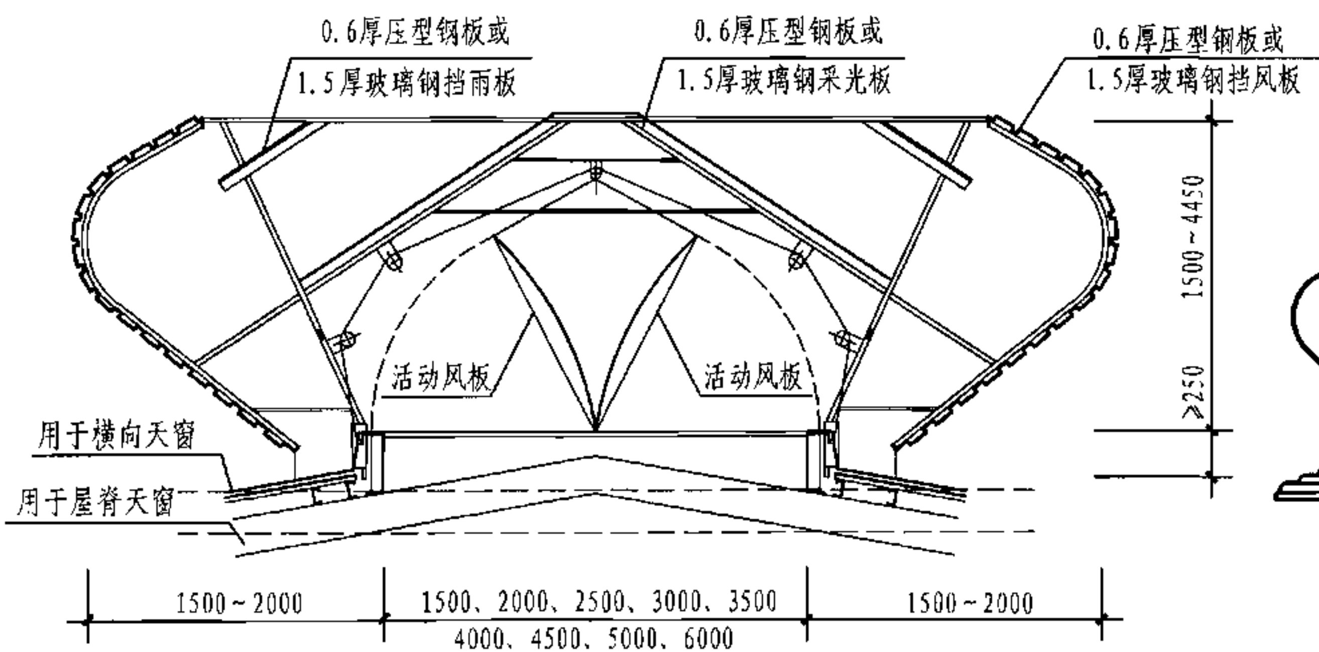
剖面图
