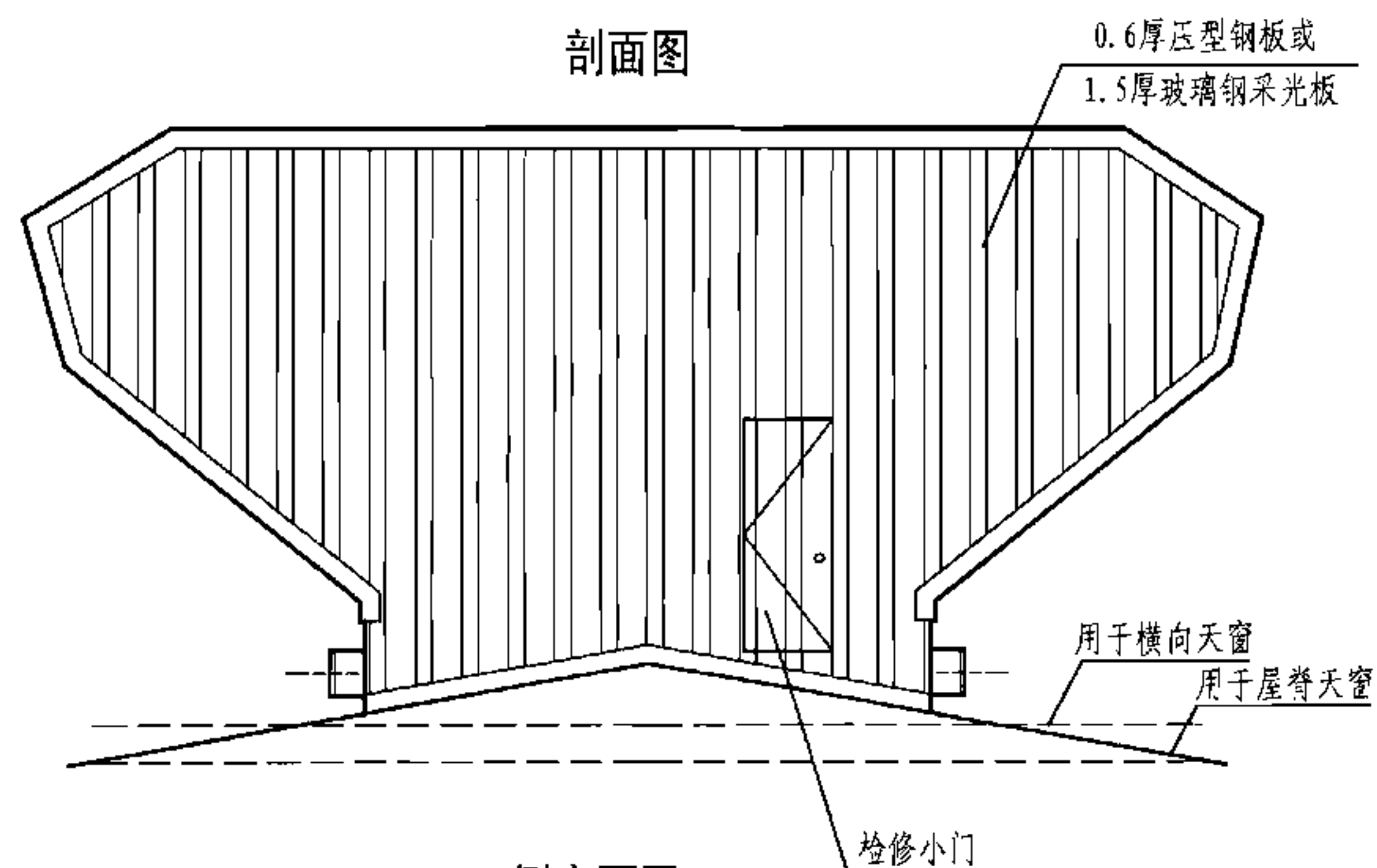
侧立面图
