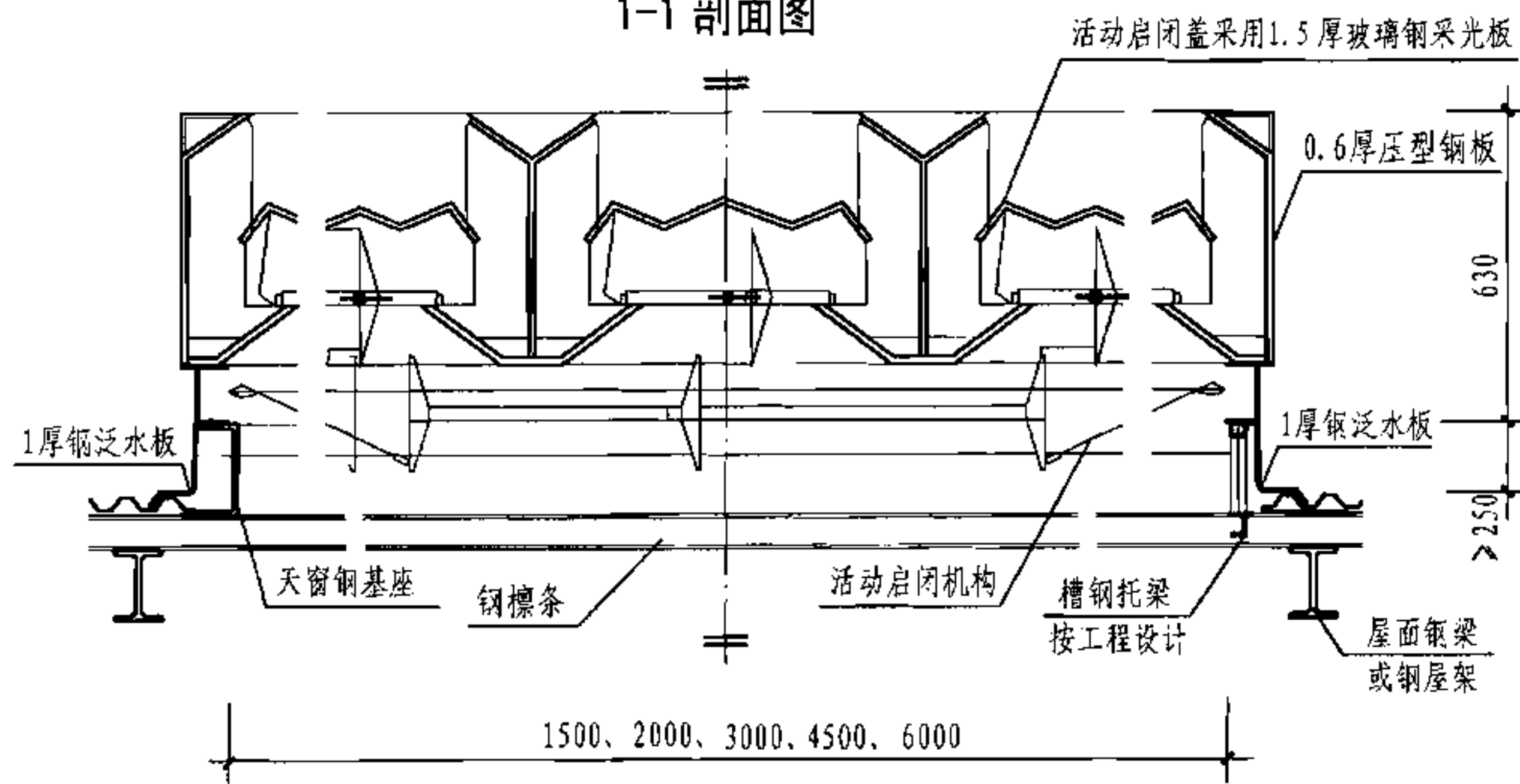
2-2 剖面图
