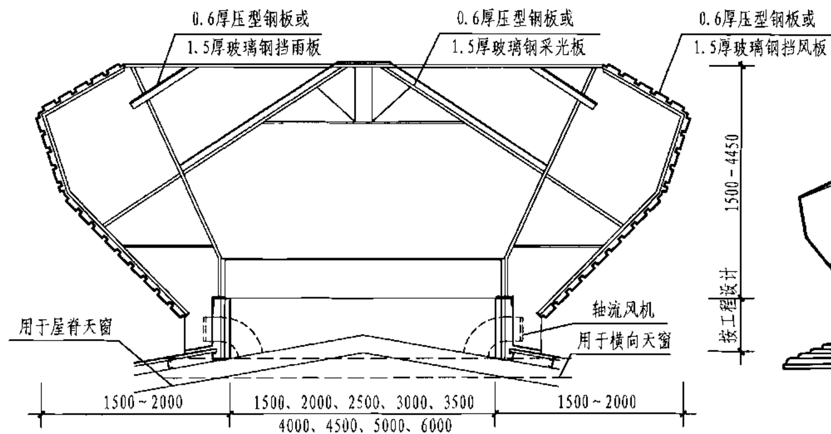
剖面图
