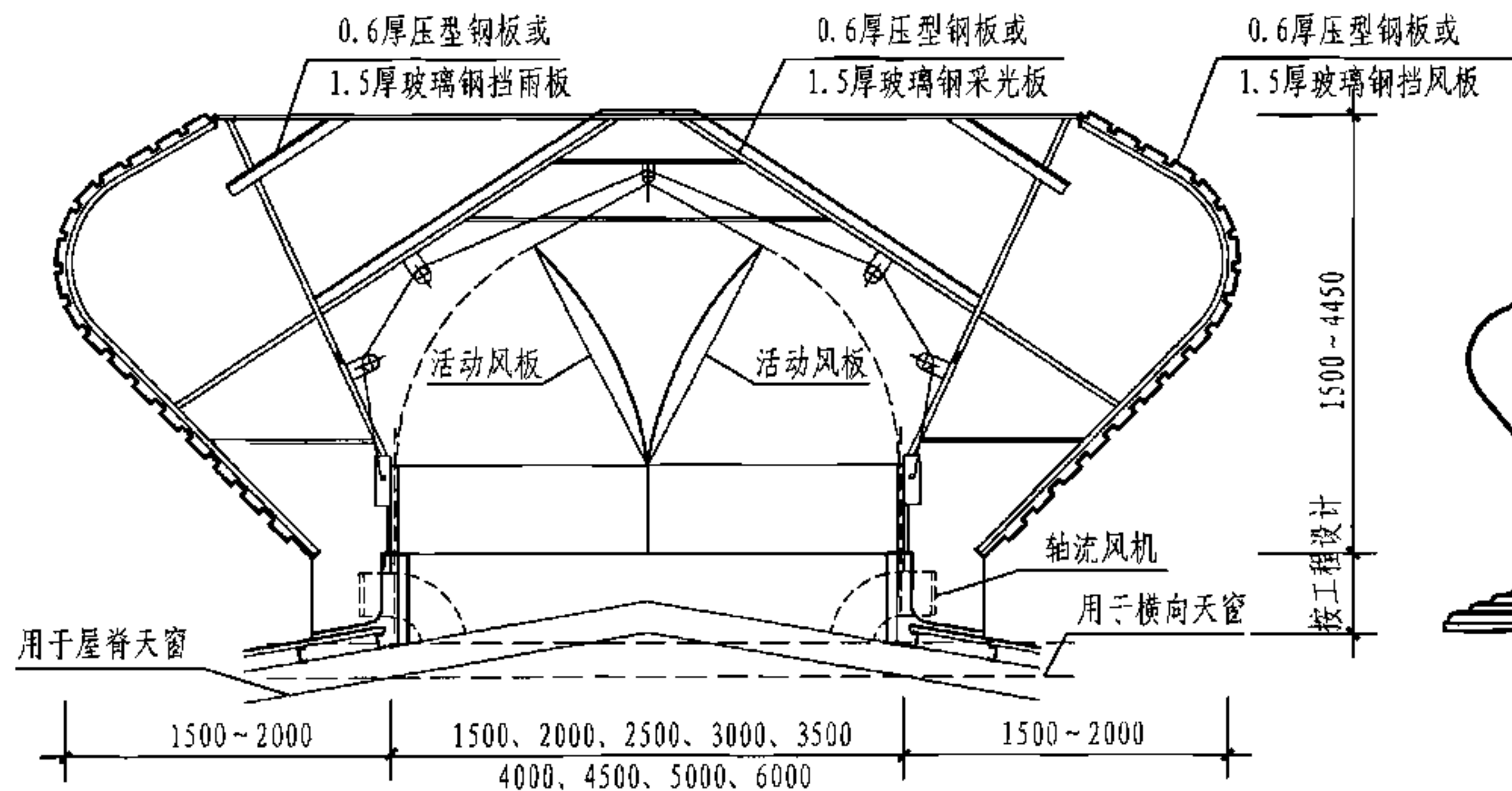
剖面图
