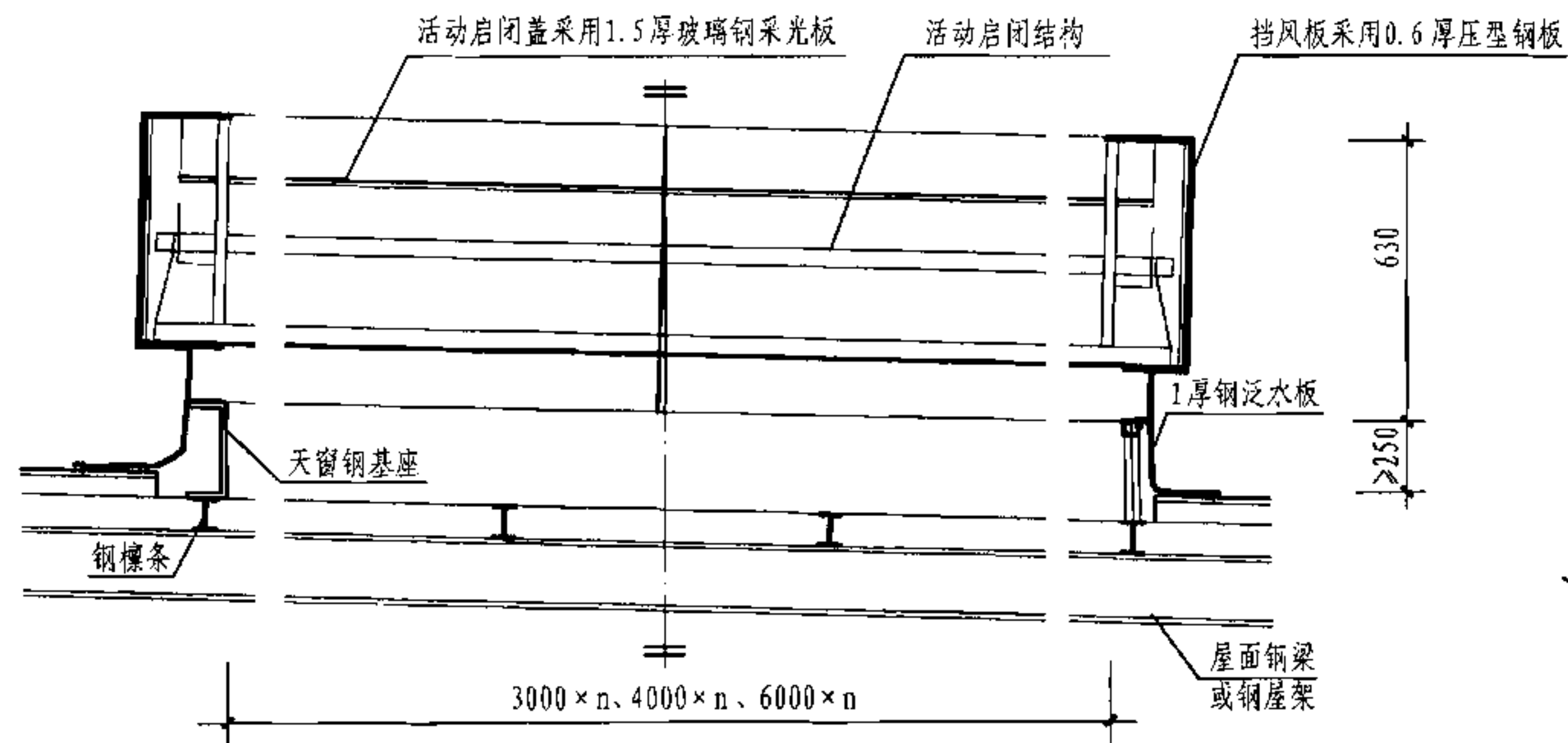
1-1 剖面图
