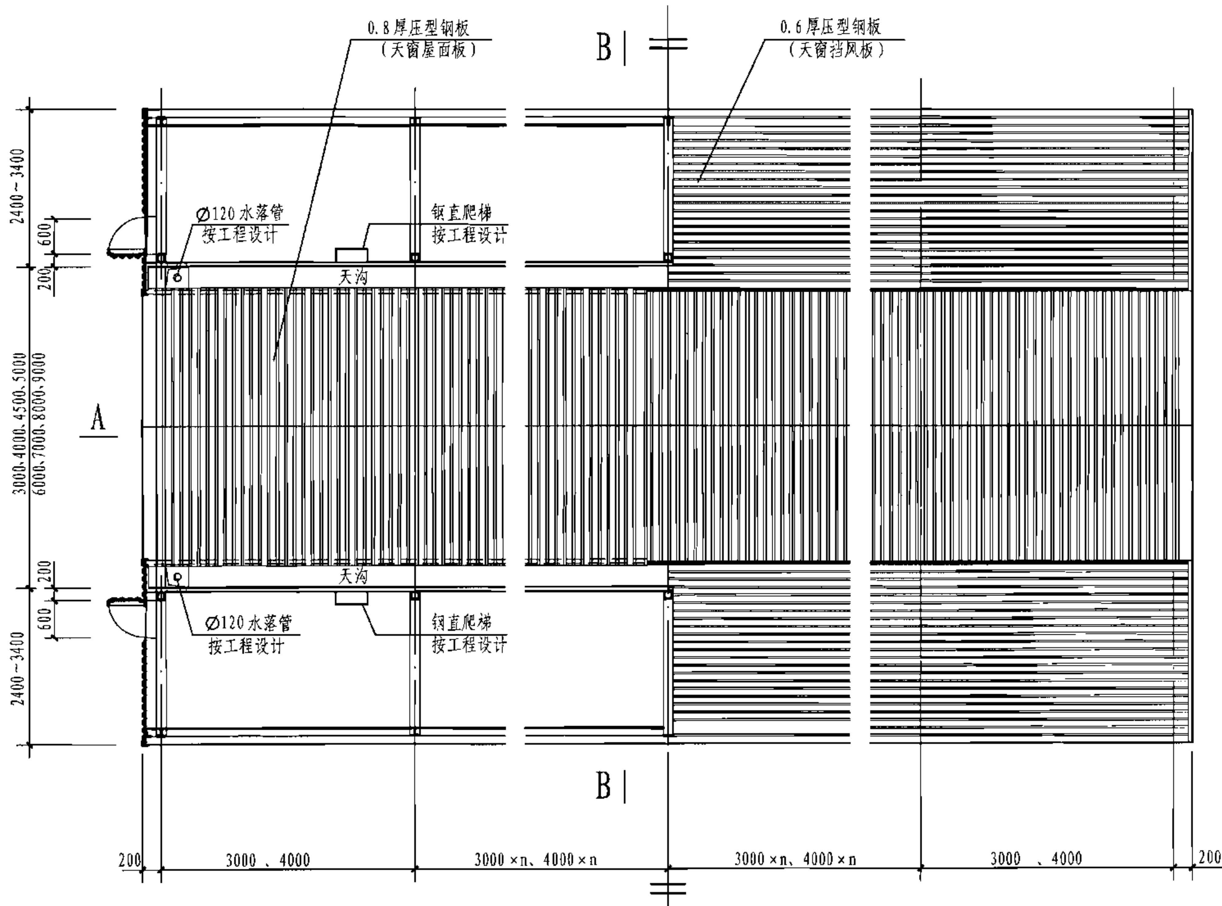
天窗平面图
