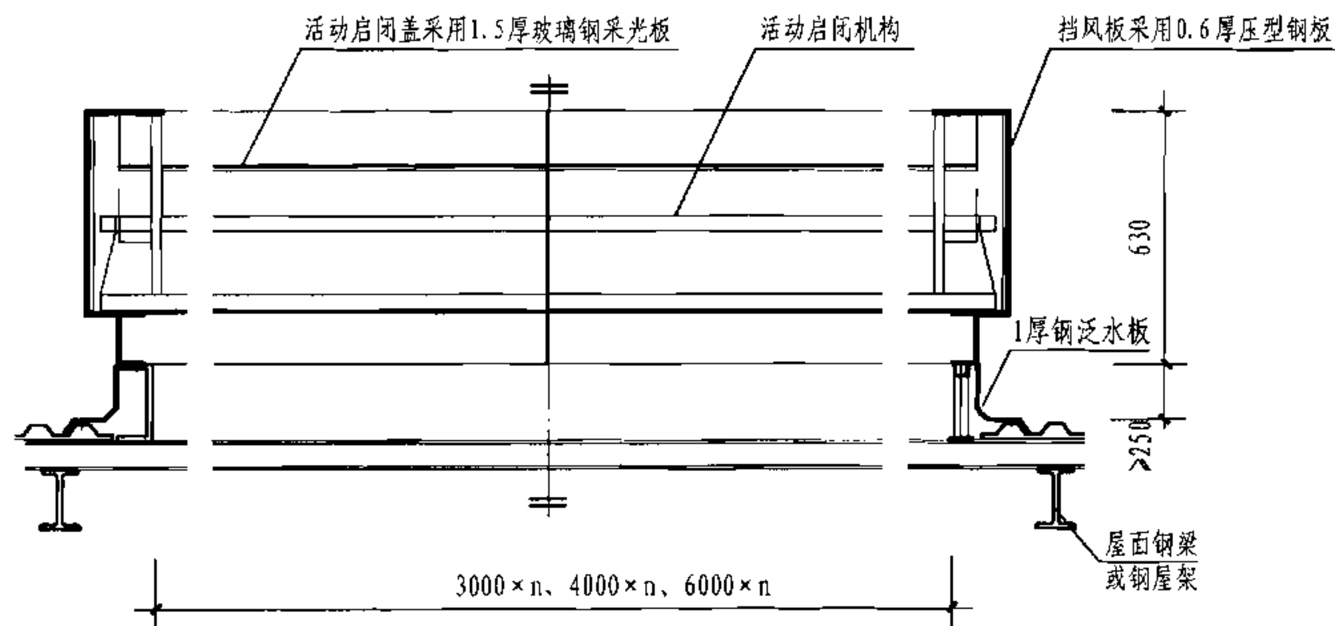
1-1 剖面图
