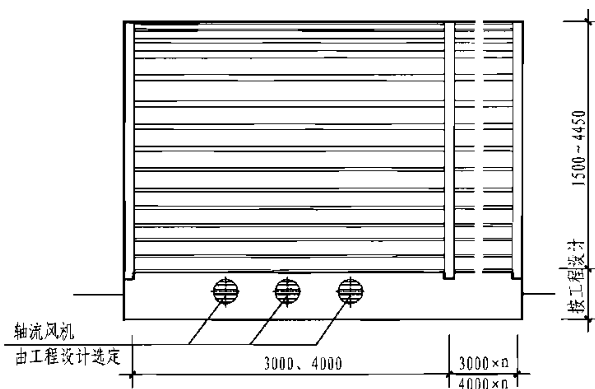
立面图
