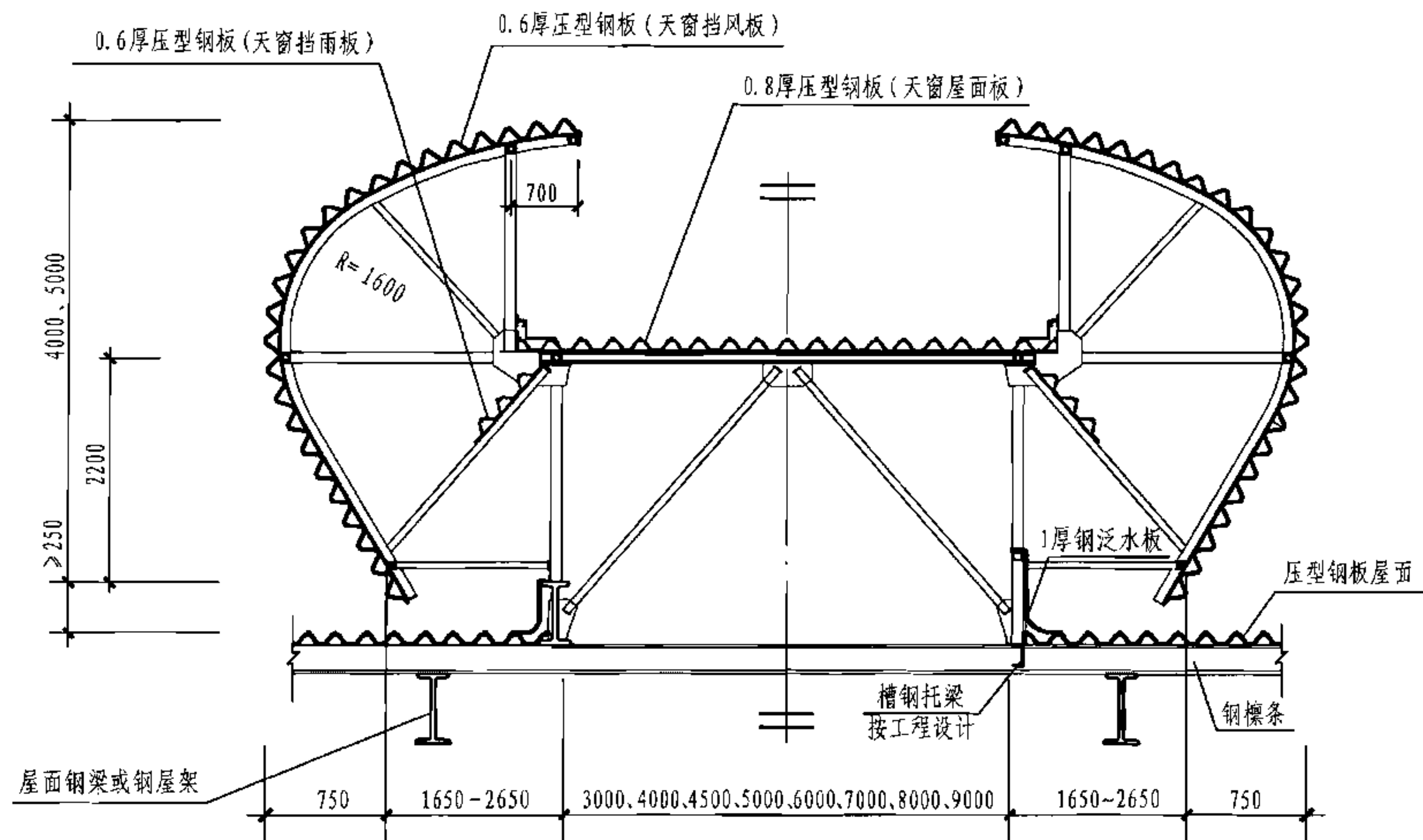
B-B 剖面图
