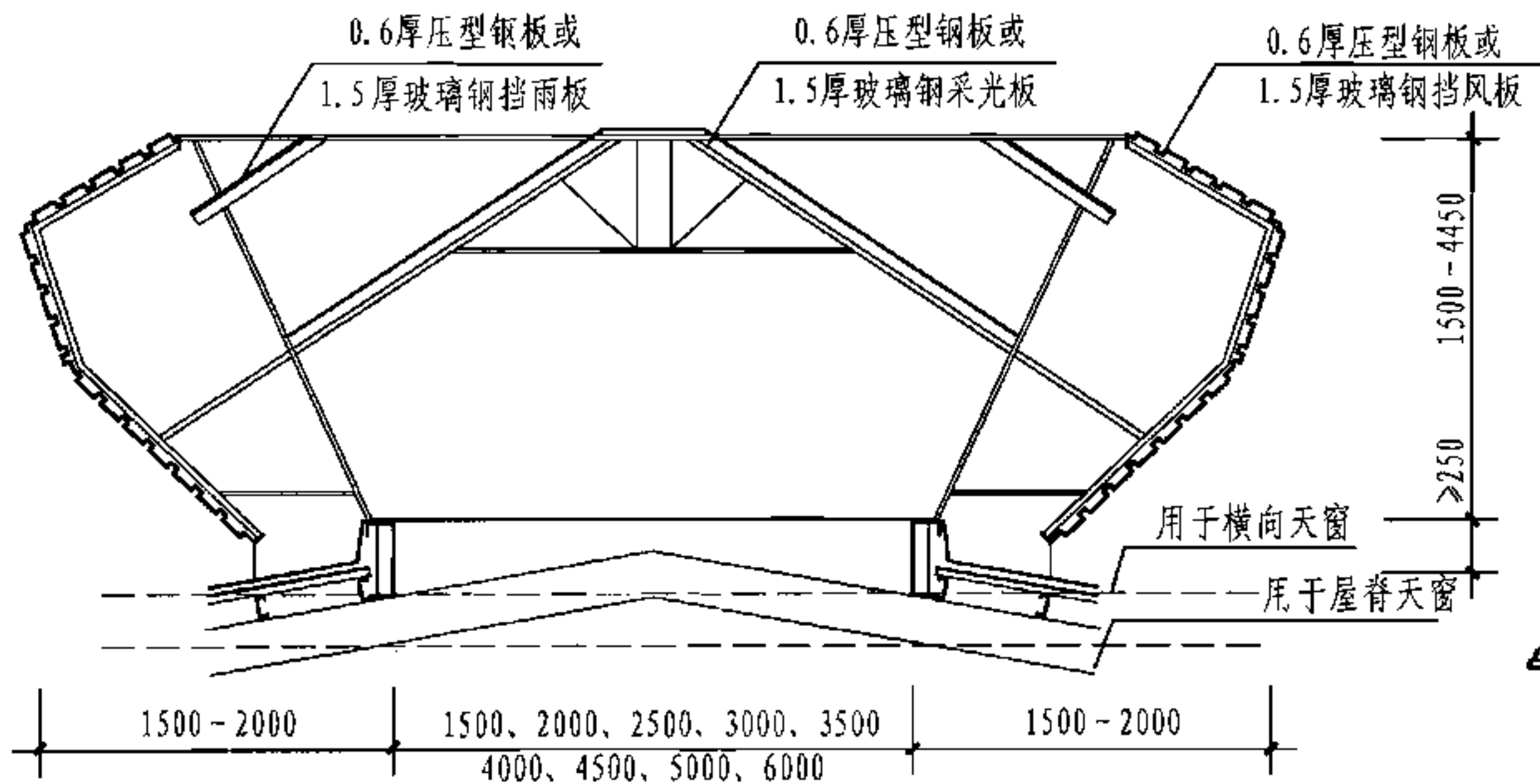
剖面图
