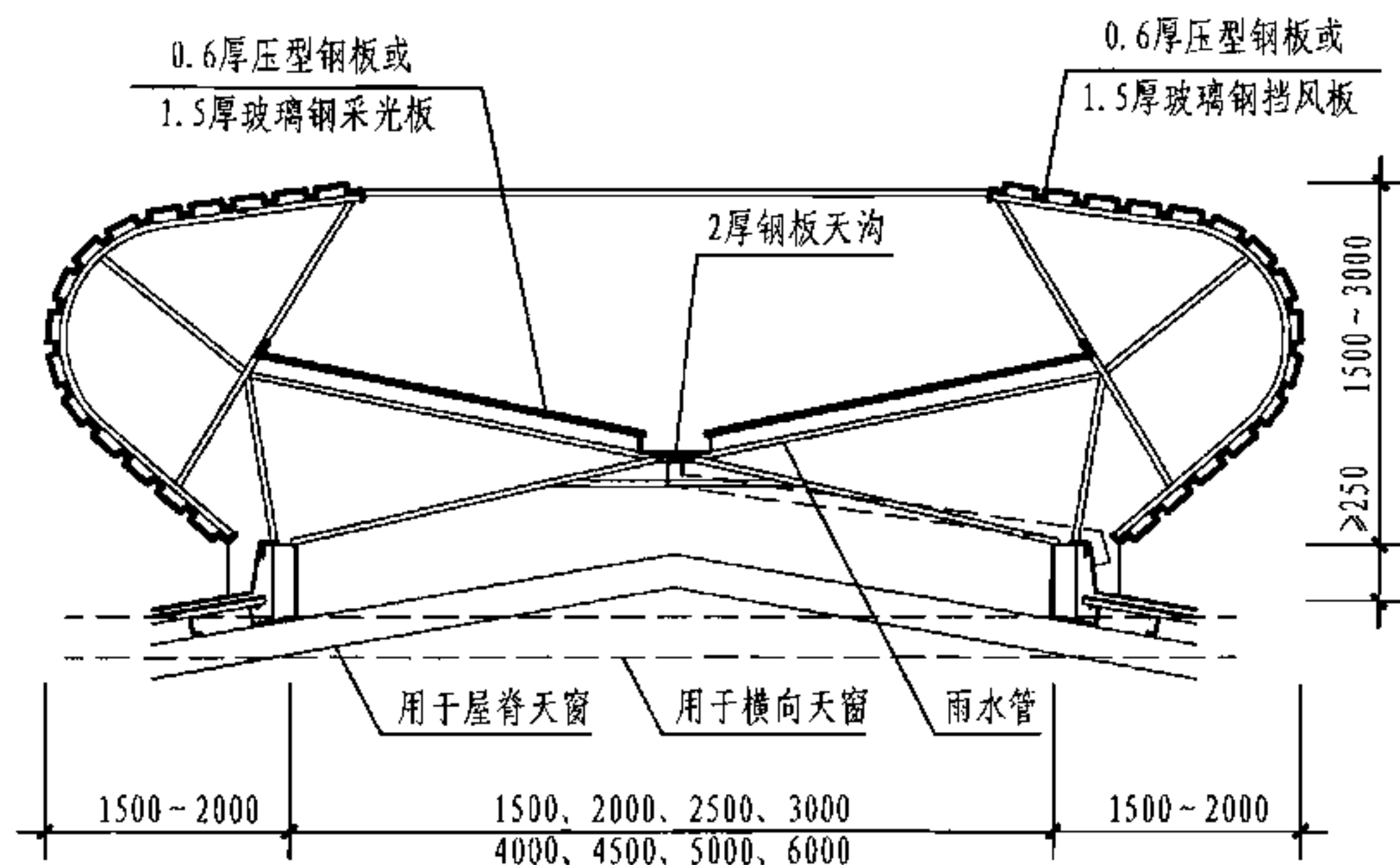
剖面图
