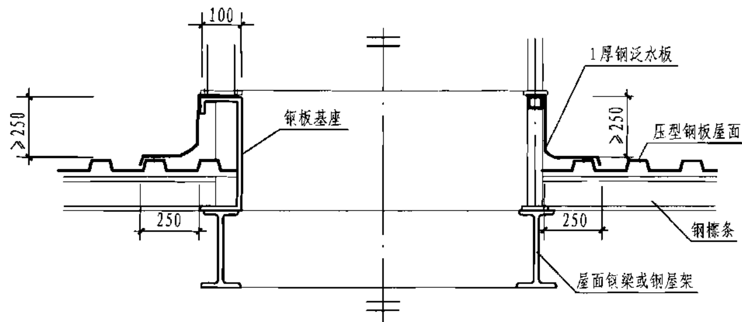
2-2 剖面图
