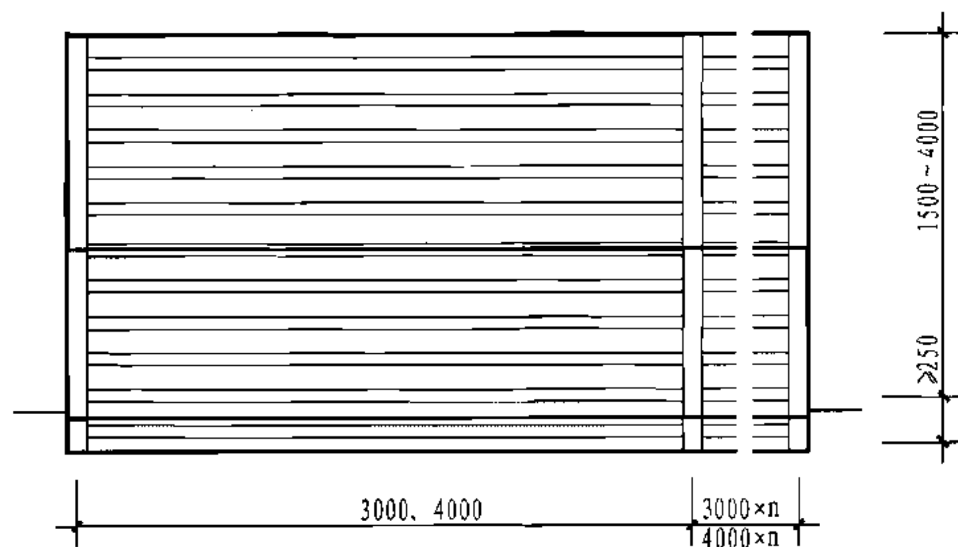
立面图
