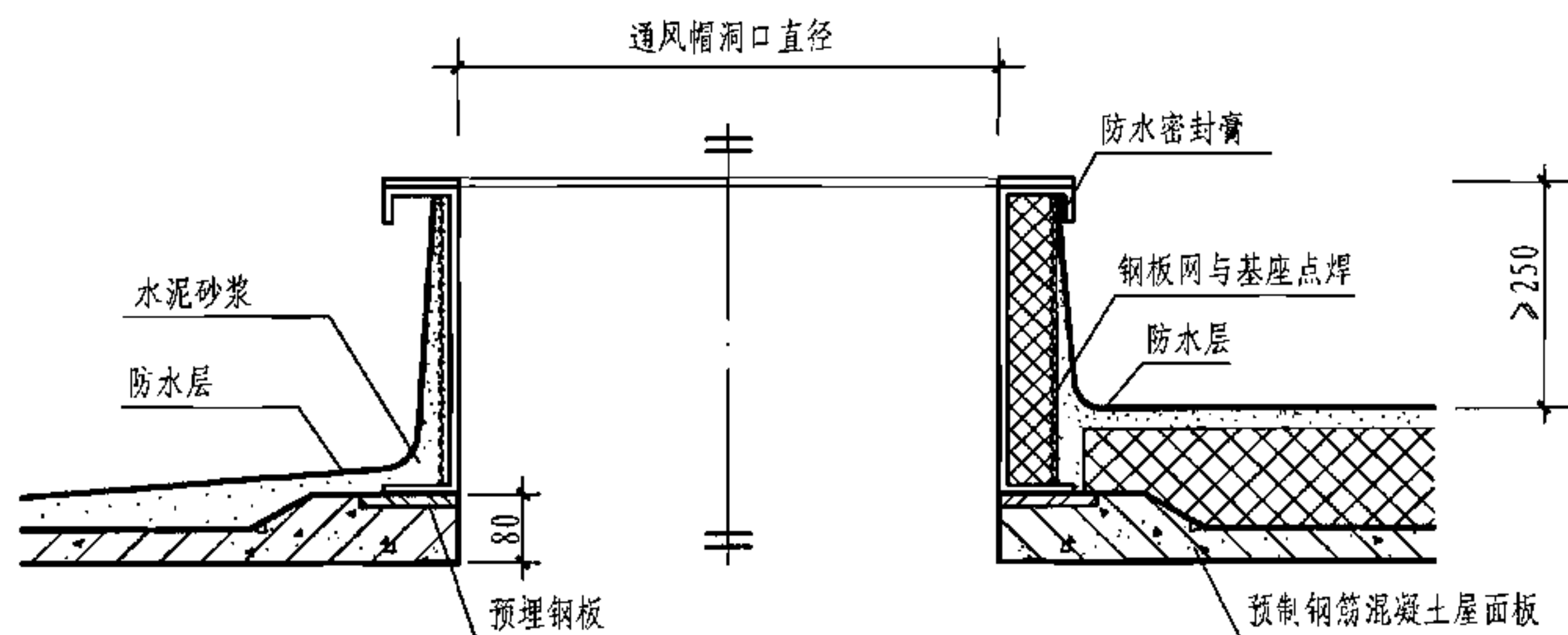
2-2剖面图
