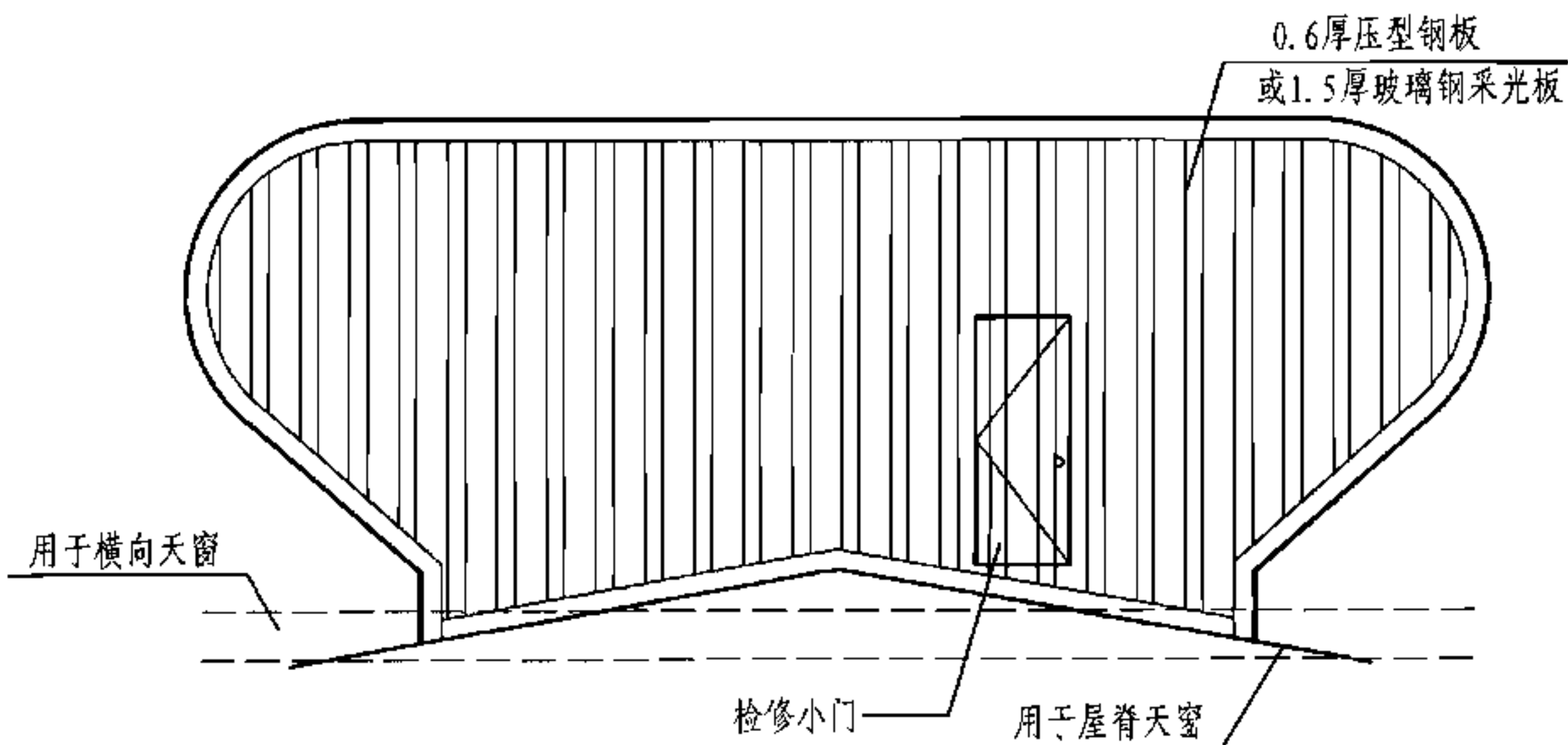
侧立面图
