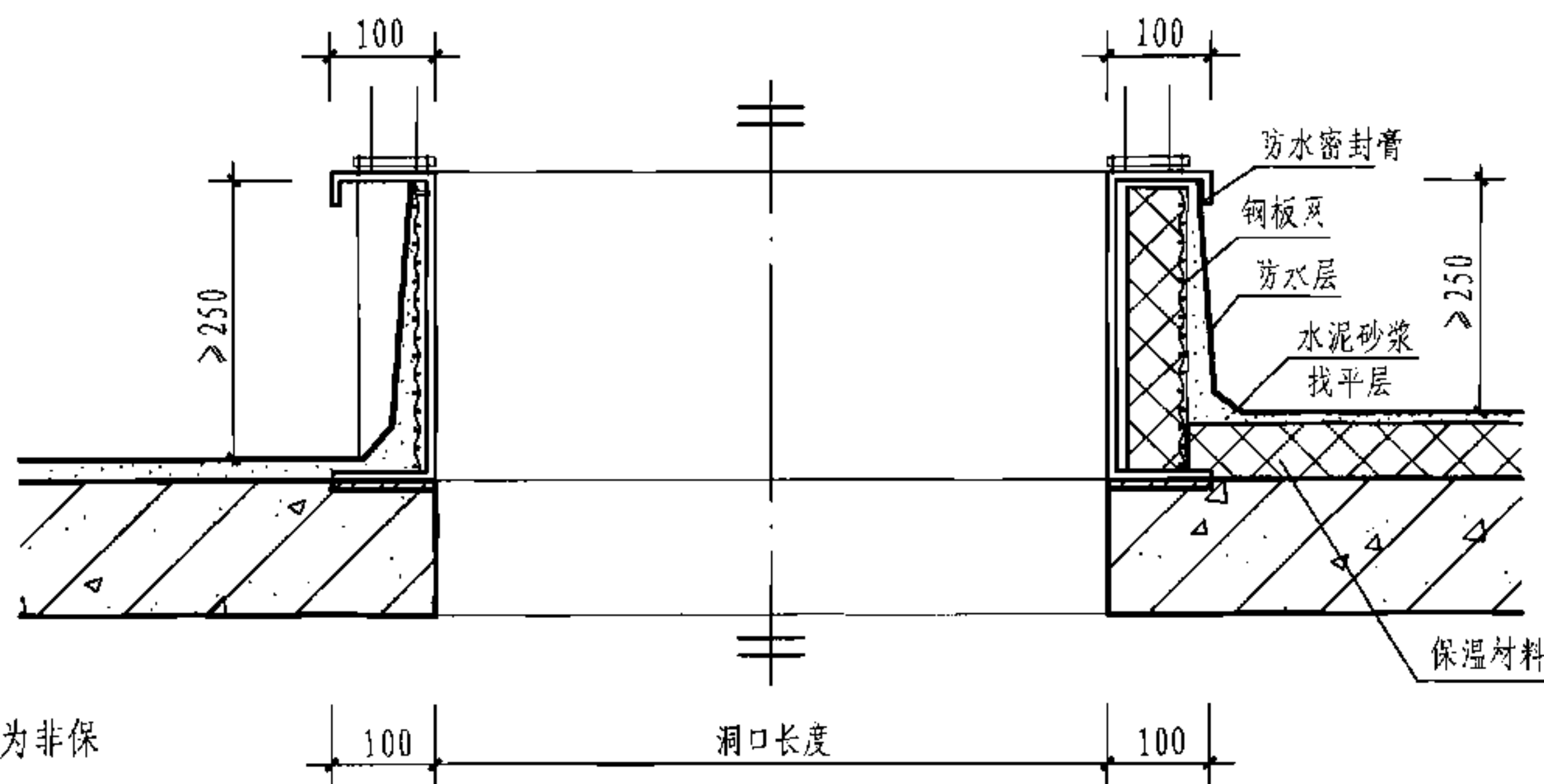
2-2 剖面图
