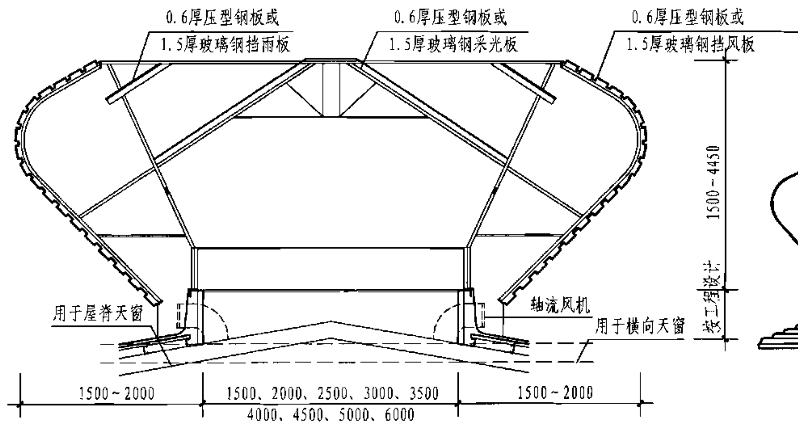
剖面图
