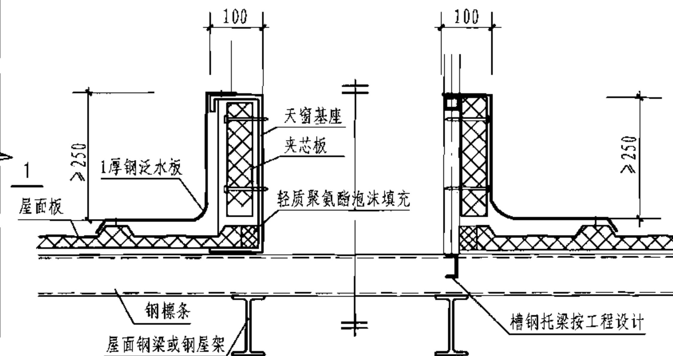
3-3 剖面图
