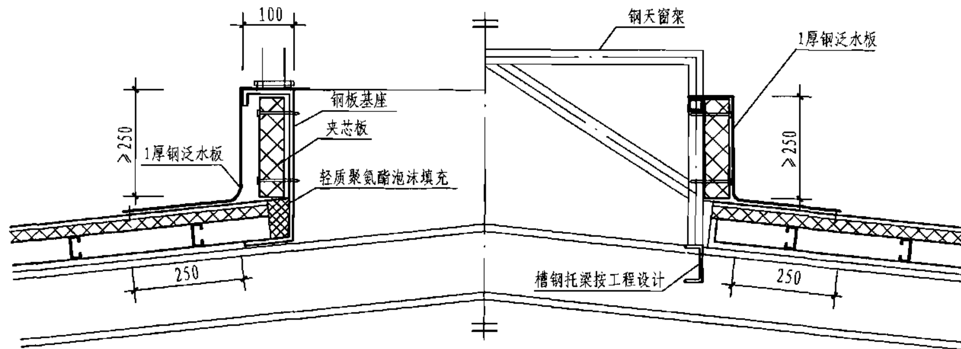
1-1 剖面图
