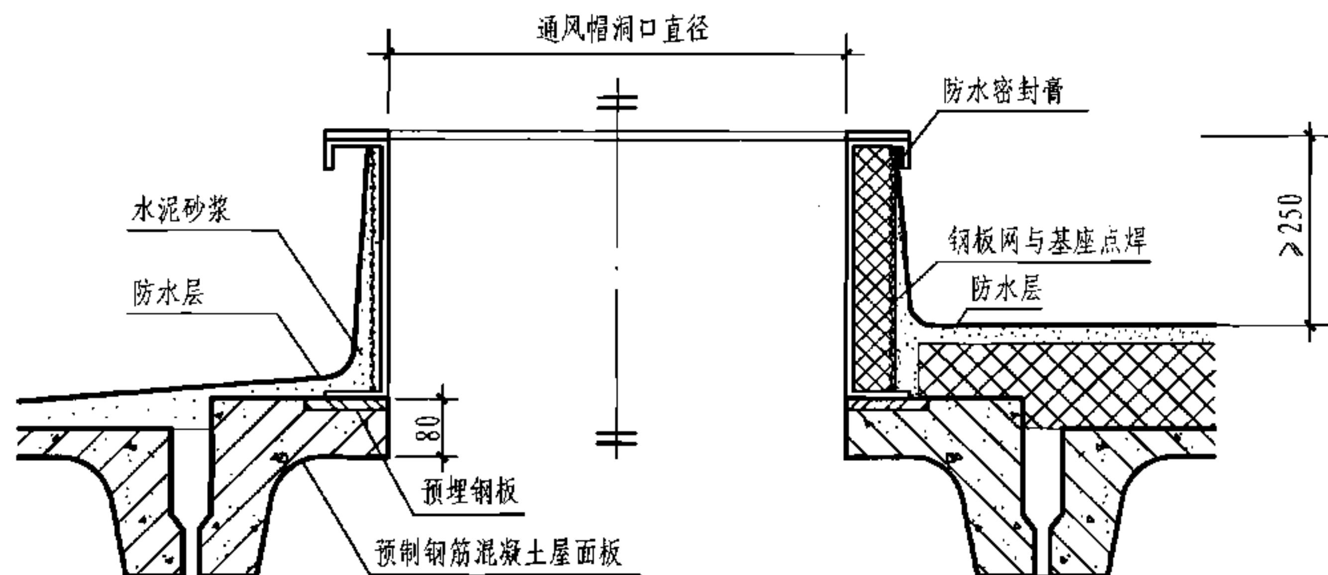
1-1剖面图
