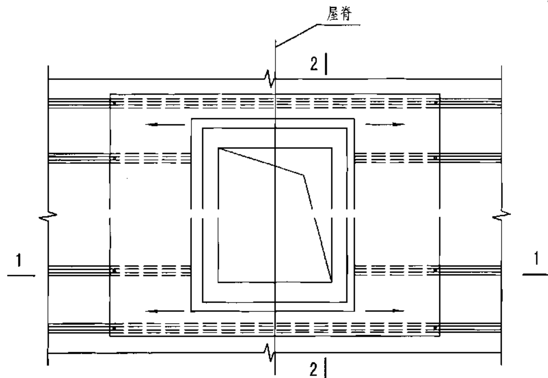
通风天窗基座洞口平面图
