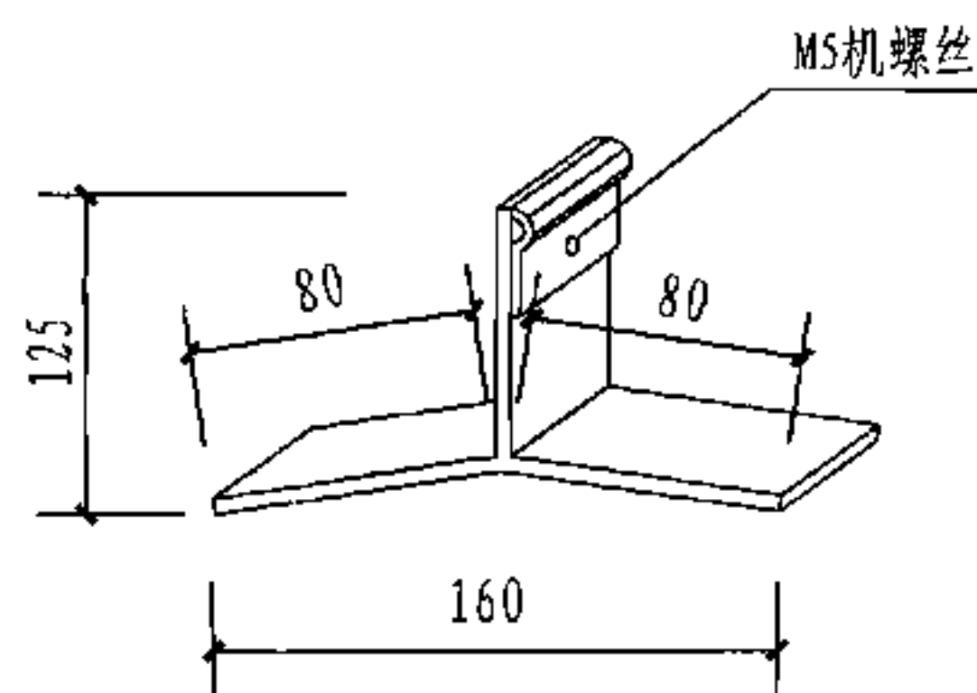
避雷带支架 ① 大样
