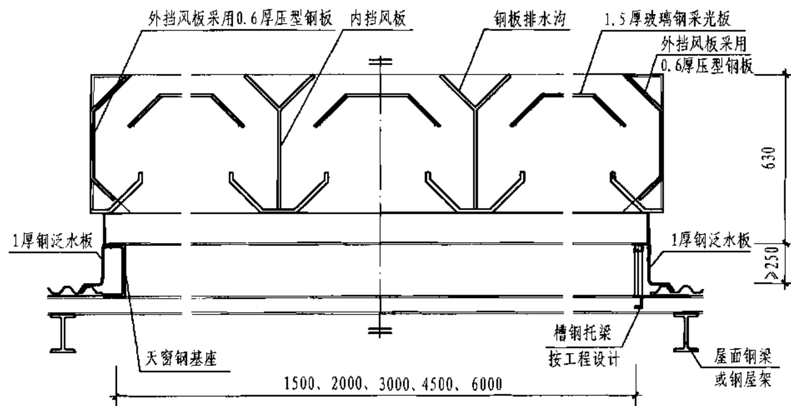
2-2 剖面图
