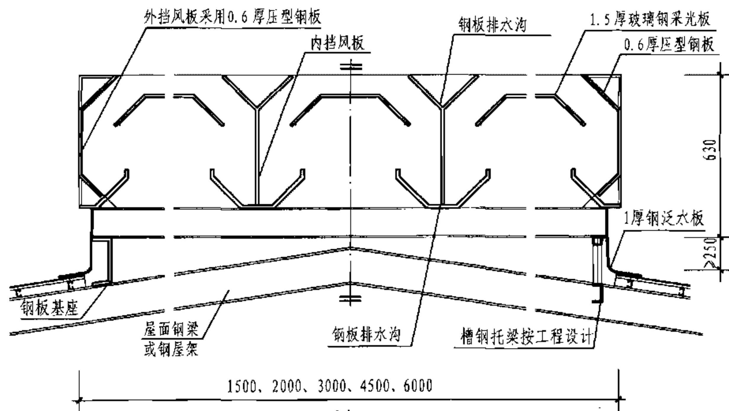
2-2 剖面图
