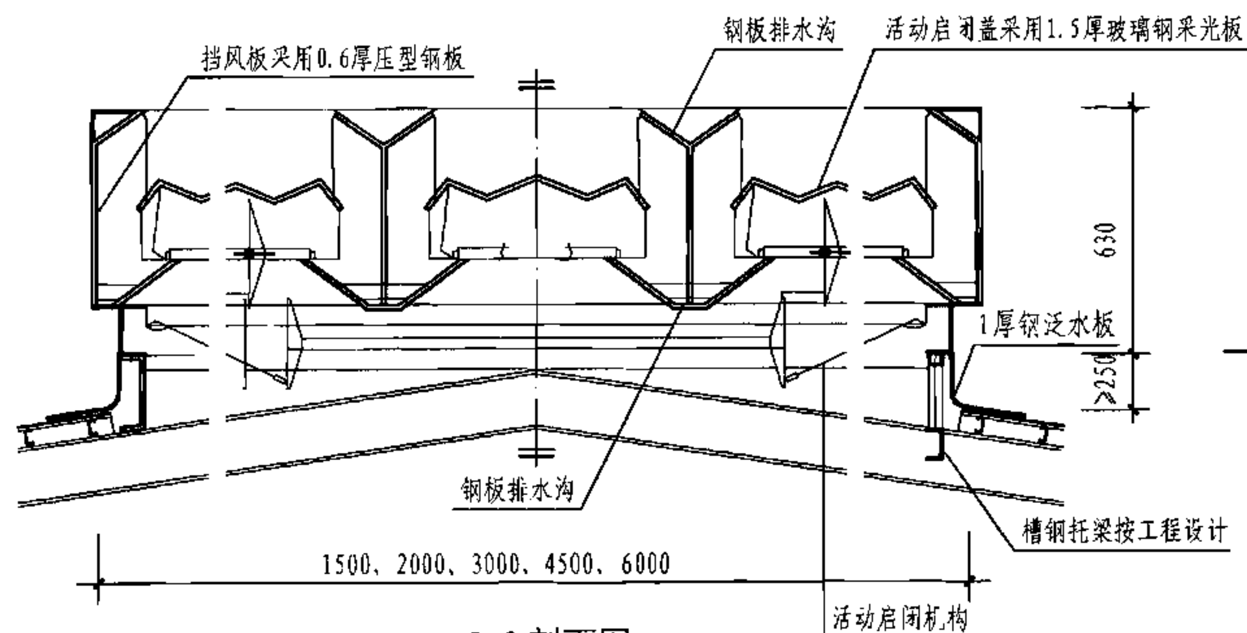
2-2 剖面图
