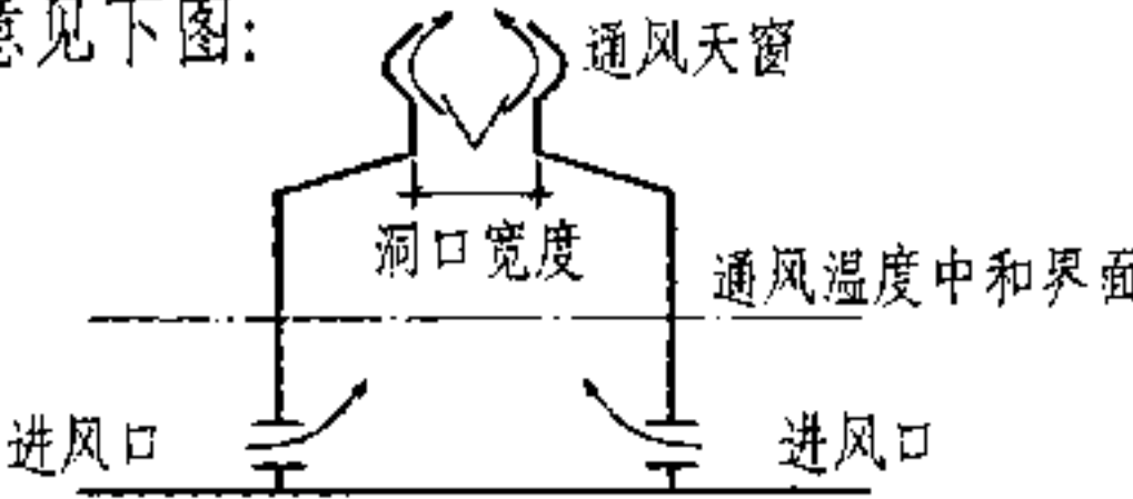
通风天窗工作原理示意图
