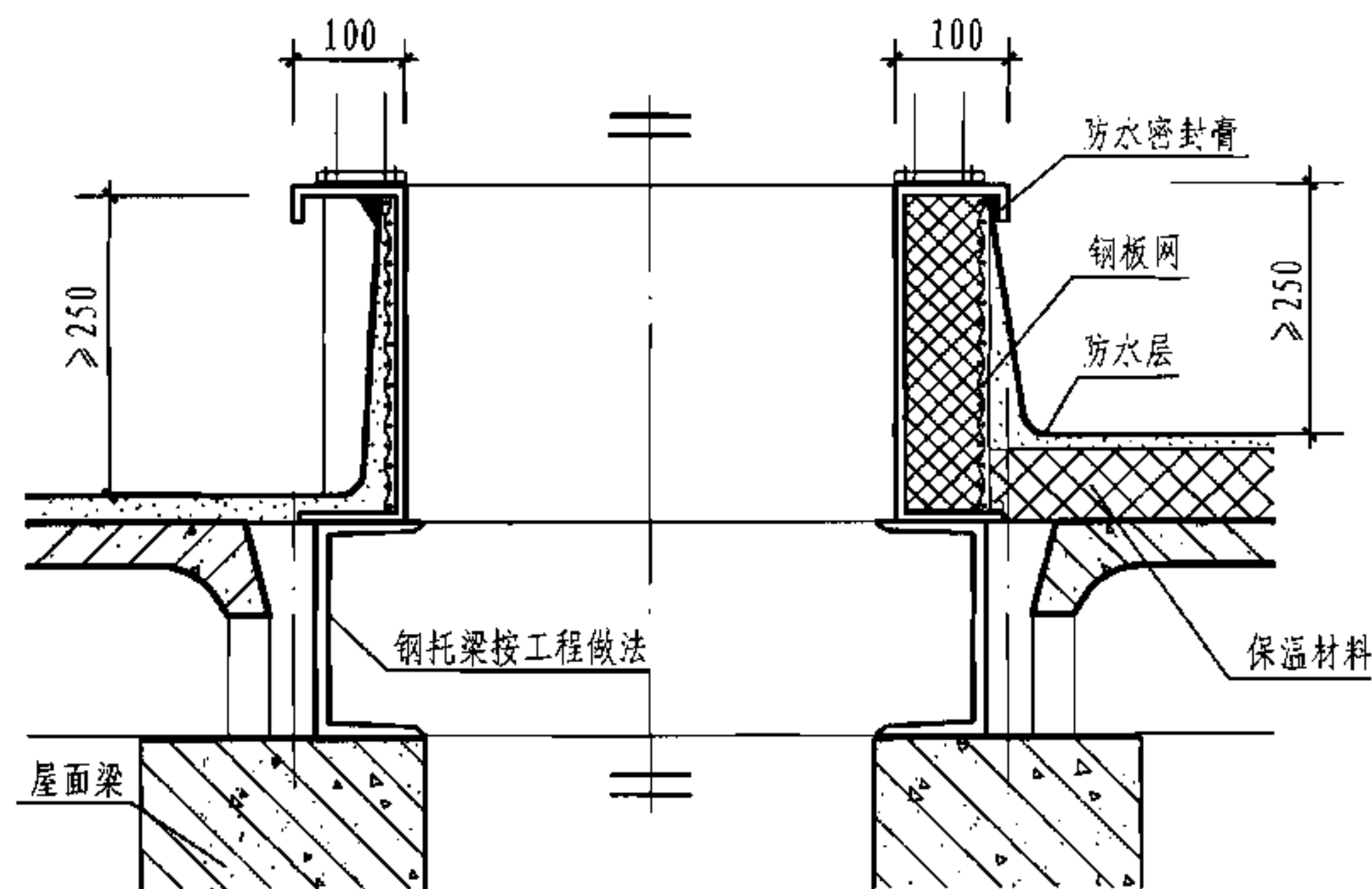
2-2 剖面图
