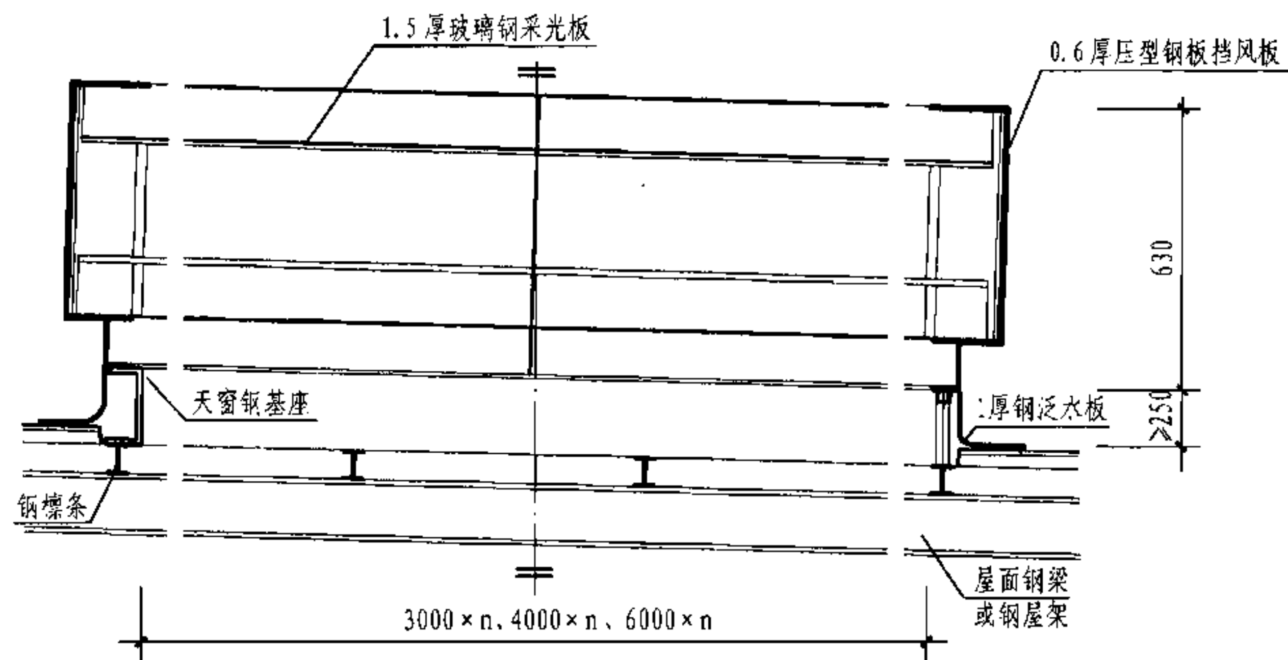
1-1 剖面图
