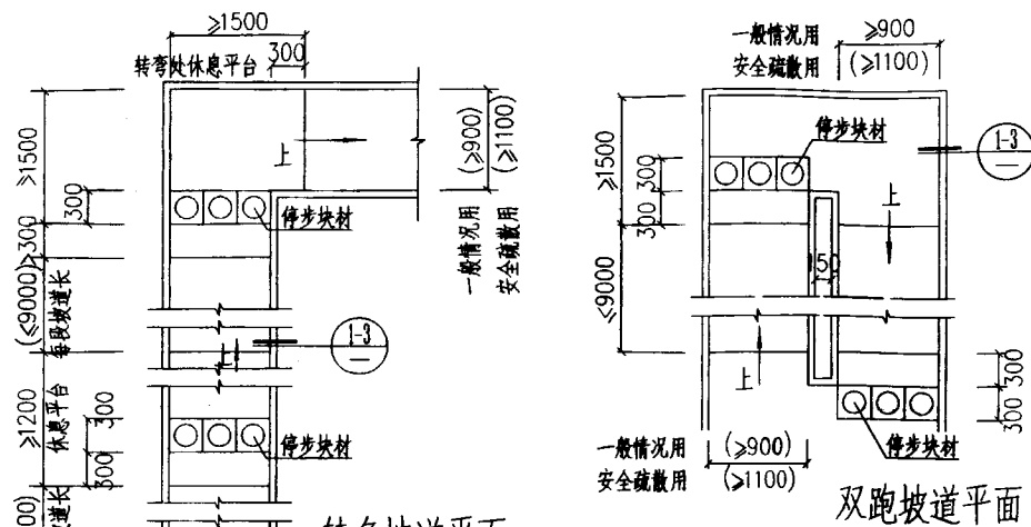
转角坡道平面
