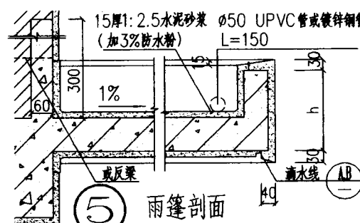
③ 雨篷剖面
