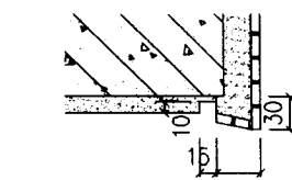
③ 滴水线 用于贴面砖
