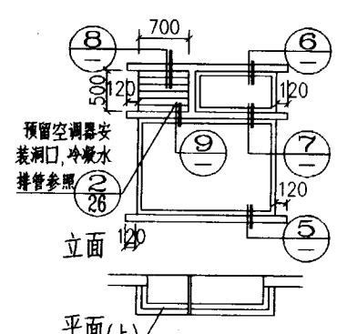
窗套示意 铝合金百页窗
