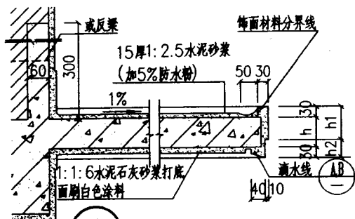
① 雨篷剖面
