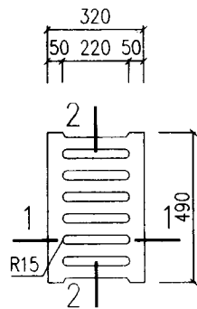
盖板平面
