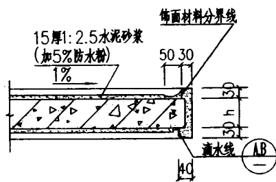
② 雨篷剖面
