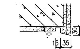
① 滴水线 用于粉刷涂料
