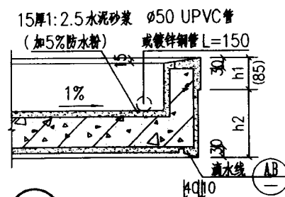
④ 雨篷剖面
