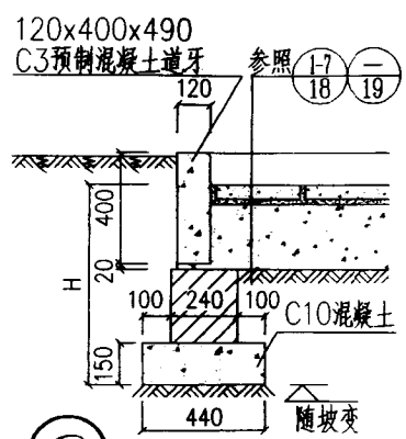
⑥ 预制混凝土道牙 用于单面坡或全宽式缘石坡道
