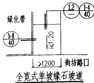
单面坡缘石坡道
