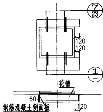
帶花槽的窗台示意
