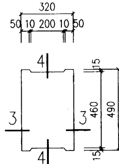
盖板平面
