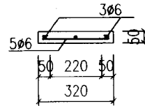
3—3 盖板剖面
