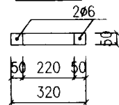
1—1 盖板断面
