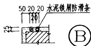
防滑条 用于水磨石、抹水泥面
