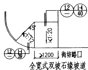
三面坡缘石坡道
