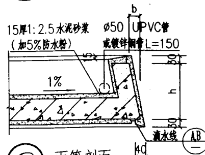
⑥ 雨篷剖面
