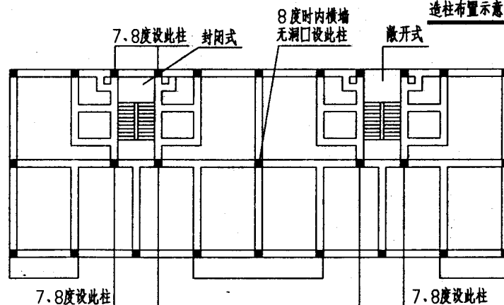
构造柱布置示意图 3
