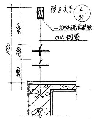
I-I 1:10
