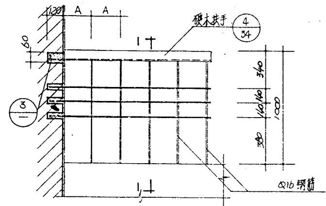
平台栏杆 1:20
