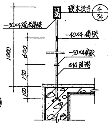
I—I 1:20
