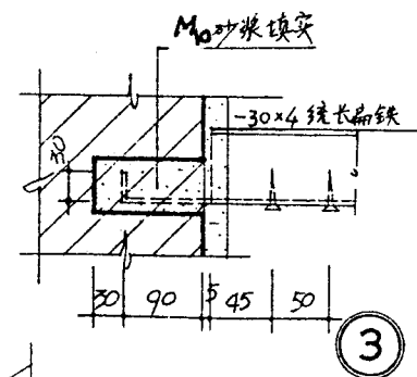
平台栏杆 1:20
