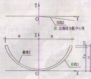
YMB纵向、横向曲线座标值
