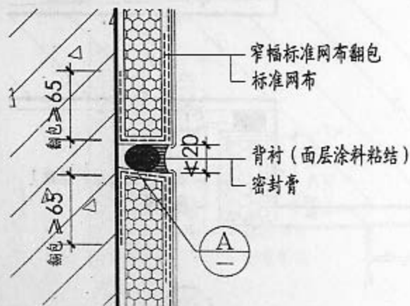
② 水平缝一般型
