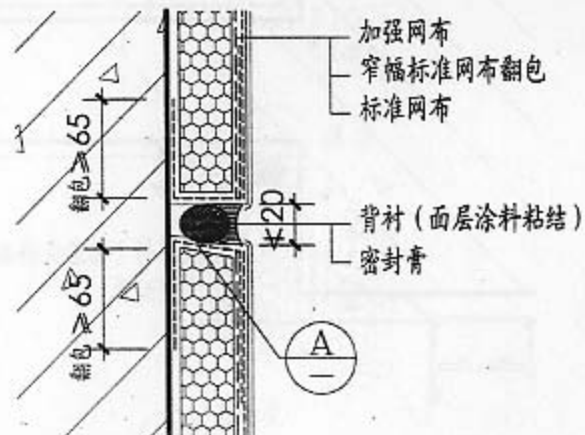
④ 水平缝加强型
