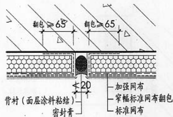
③ 垂直缝加强型
