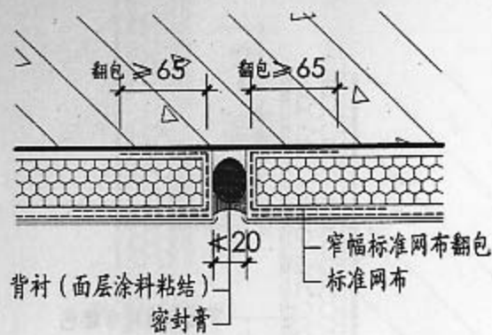
① 垂直缝一般型
