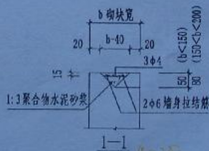
拉结筋连接
