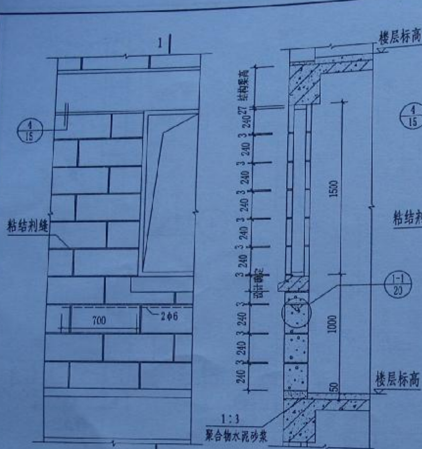
砌筑立面排块示意图 A (窗高 1.5m 窗台 1.0m)
