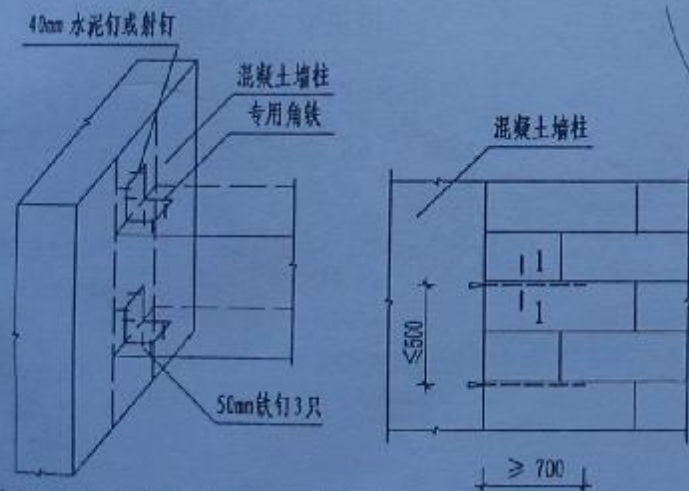
填充墙和混凝土墙柱专用角铁连接 拉结筋详图
