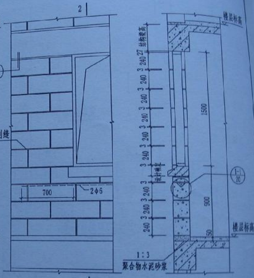
砌筑立面排块示意图 B (窗高 1.5m 窗台 0.9m)
