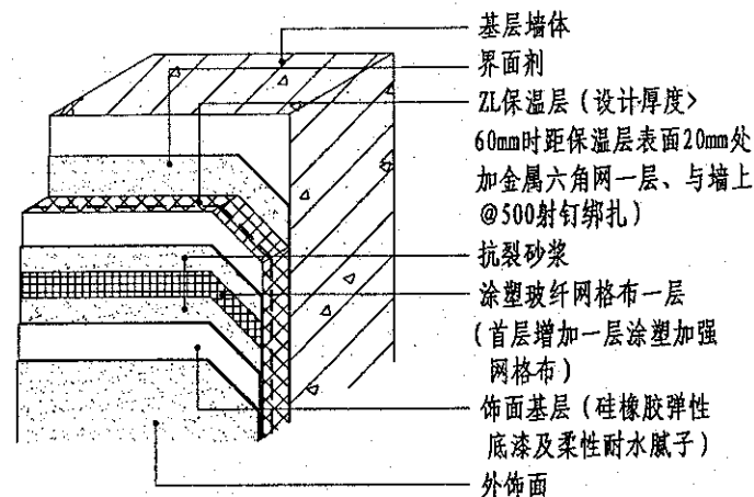
保温层做法示意图 (B)
