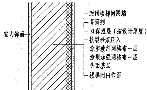
④ 封闭楼梯间隔墙
