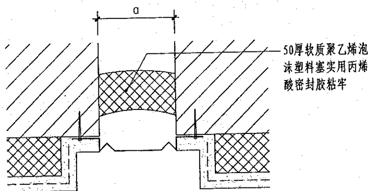
② 外墙变形缝 (二)
