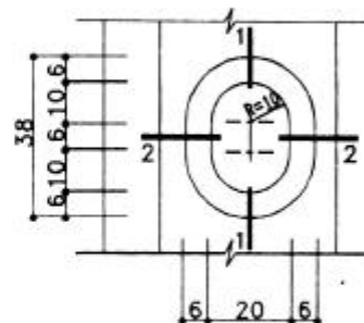
锁舌孔立面
