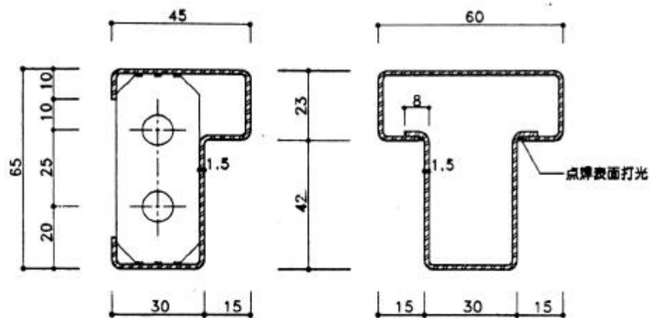
钢板折弯型材用于40厚门扇
