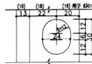
门框开孔位置,尺寸
