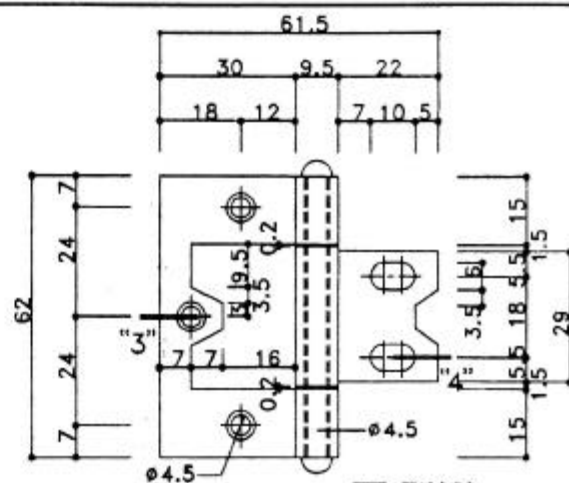
IV 型铰链
