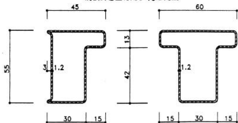
钢板折弯型材用于40厚门扇
