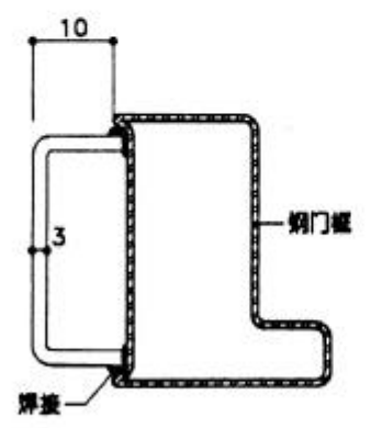
铁脚焊接位置图
