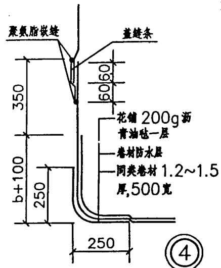
卷材转角接槎做法 (括号内数字用于合成高分子类卷材)
