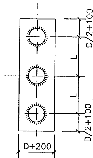
③ 三管
