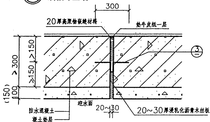
② 底板 (括号内数字用于软土层)
