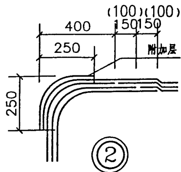
卷材转角甩槎做法 (括号内数字用合成高分子类卷材)
