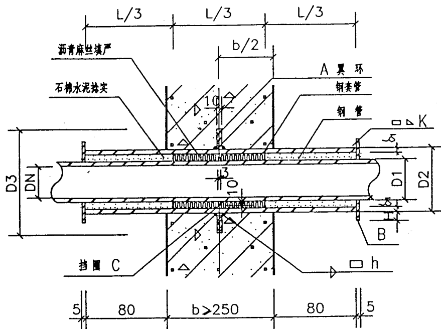
预埋钢套刚性接法 (适用于钢管)
