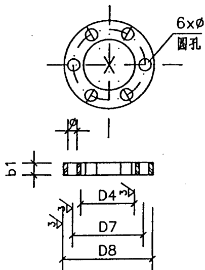
⑦ 法兰盘
