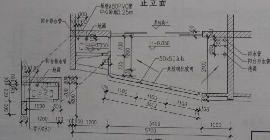
平面
