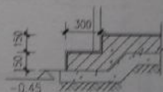
混凝土踏步
