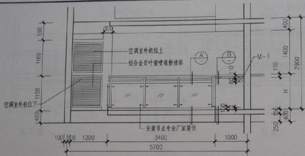
正立面
