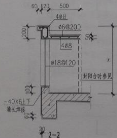
阳台平立剖面图 (二)
