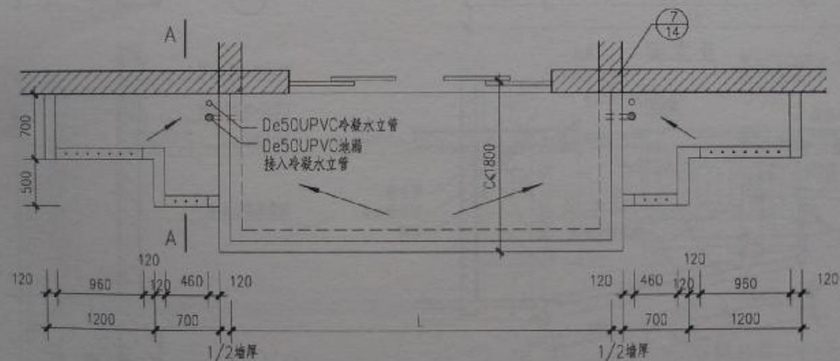
阳台和空调搁板平立剖面图(七)
