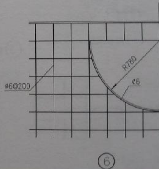
阳台节点详图 (四)
