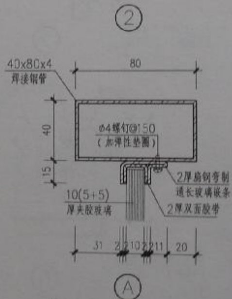
阳台节点详图 (六)
