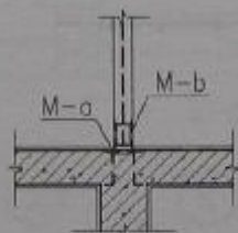
③ 阳台隔板与下梁连接
