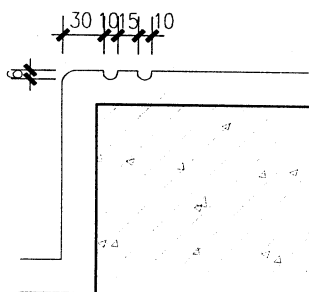
⑥ 水泥面踏步防滑条
