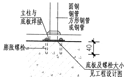
③ 膨胀螺栓锚固底板 立杆焊在地板上
