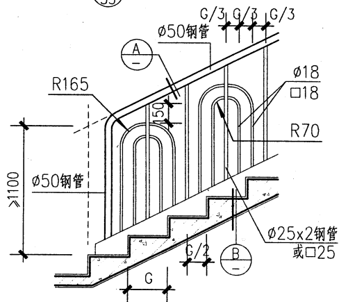
② 圆钢立柱 ③ 方钢立柱
