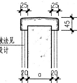
⑥ 水泥砂浆抹面扶手
