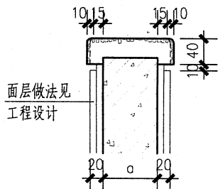
④ 水泥砂浆抹面扶手
