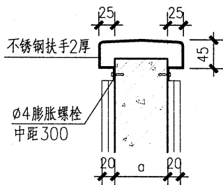
⑧ 不锈钢扶手
