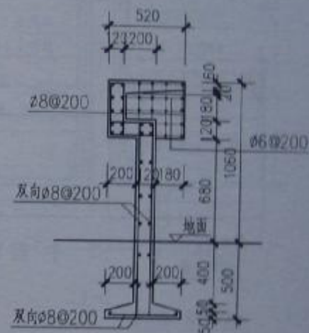
配筋图
