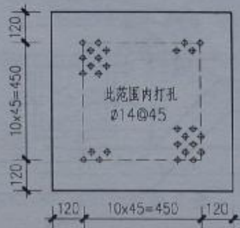
盖板平面图
