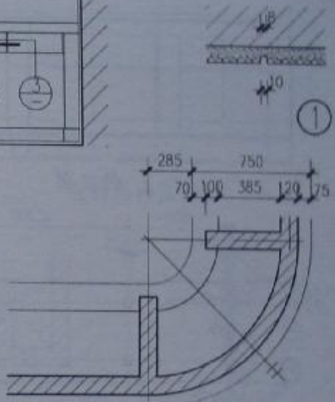
转角平面
