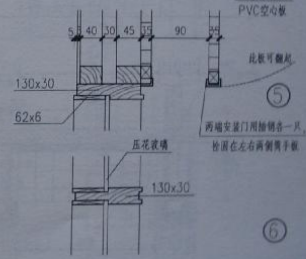
花格隔断(二)
