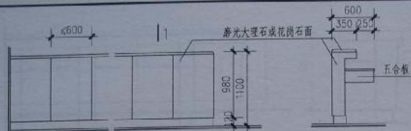
外立面 1-1
