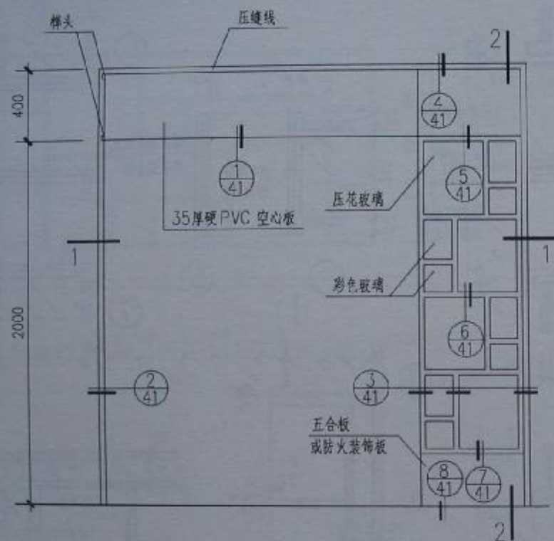
立面图
