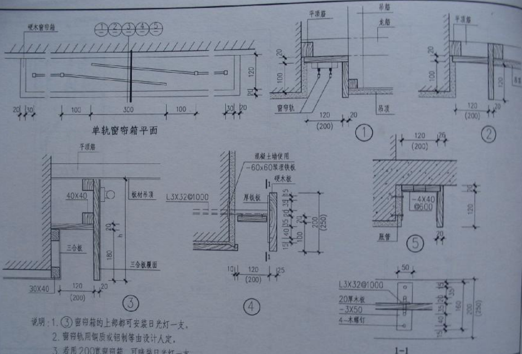
单轨窗帘箱
