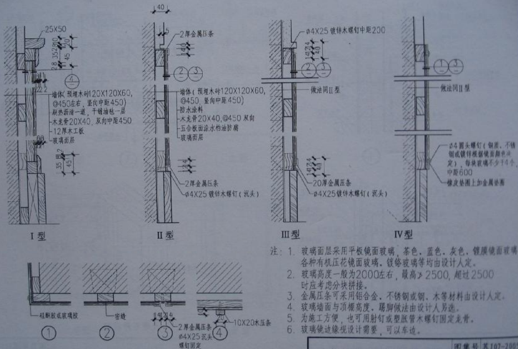
玻璃墙面、柱面(一)
