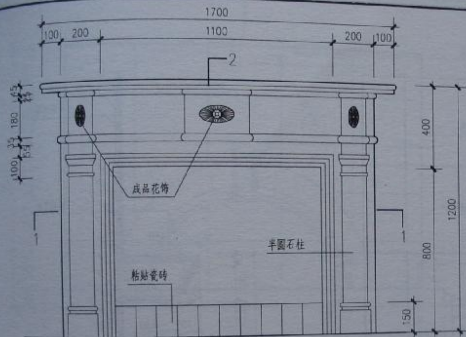
立面 2
