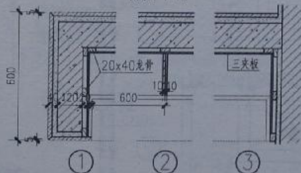
转角平面
