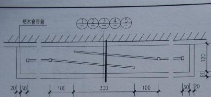
单轨窗帘箱平面
