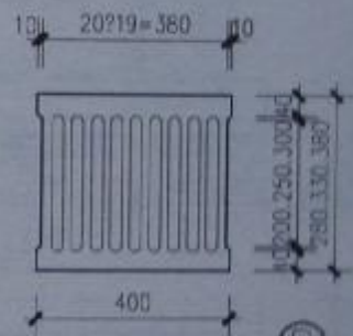
铸铁盖板
