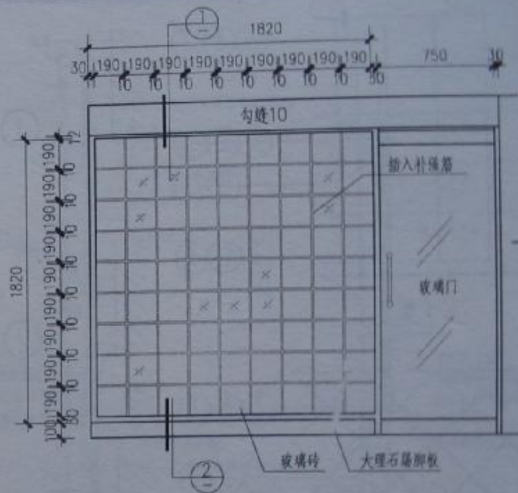
立面图
