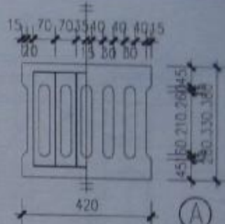
预制混凝土盖板(甲)
