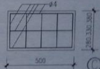
预制混凝土盖板(乙)
