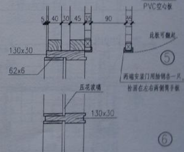
花格隔断(二)
