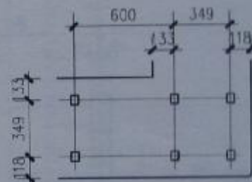
转角平面
