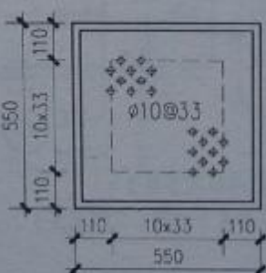
滤斗底板平面图
