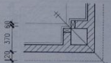
转角平面
