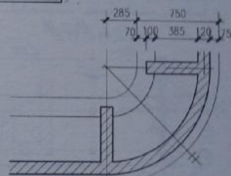
转角平面
