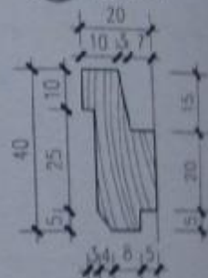
⑧ 挂镜线
