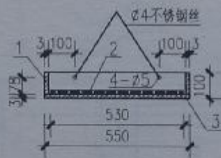
滤斗剖面图
