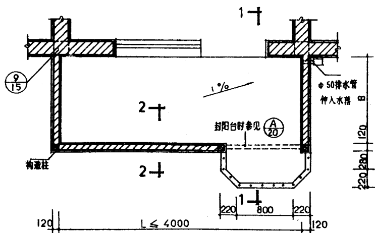
平面图
