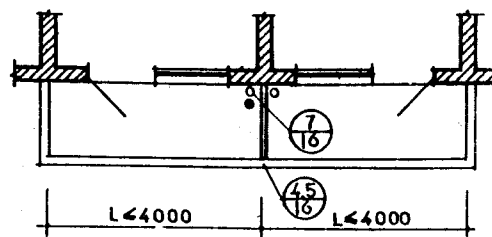
③ 双连凸阳台平面
