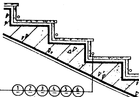
楼梯踏步剖面
