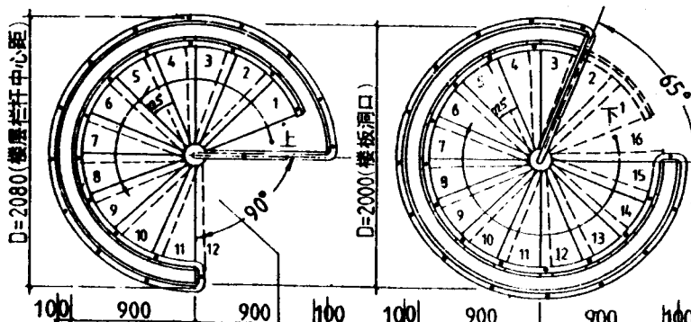
A型平面 为保证楼梯通行高度，此 楼下不可设梁（A—D型） B型平面
