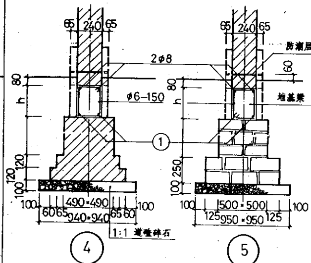
(二) 围墙独立基础
