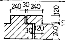
① 伸缩缝砌法
