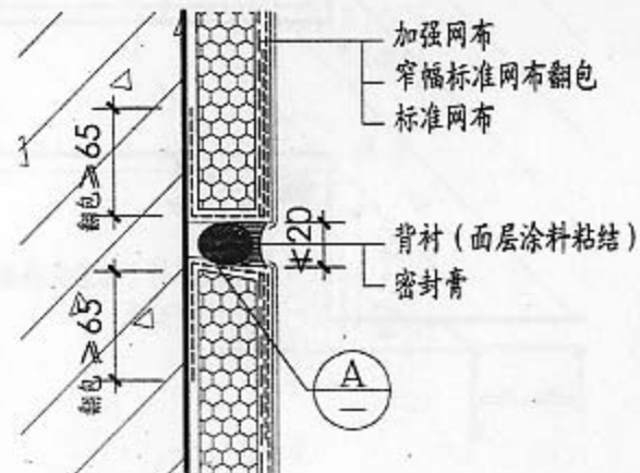
④ 水平缝加强型
