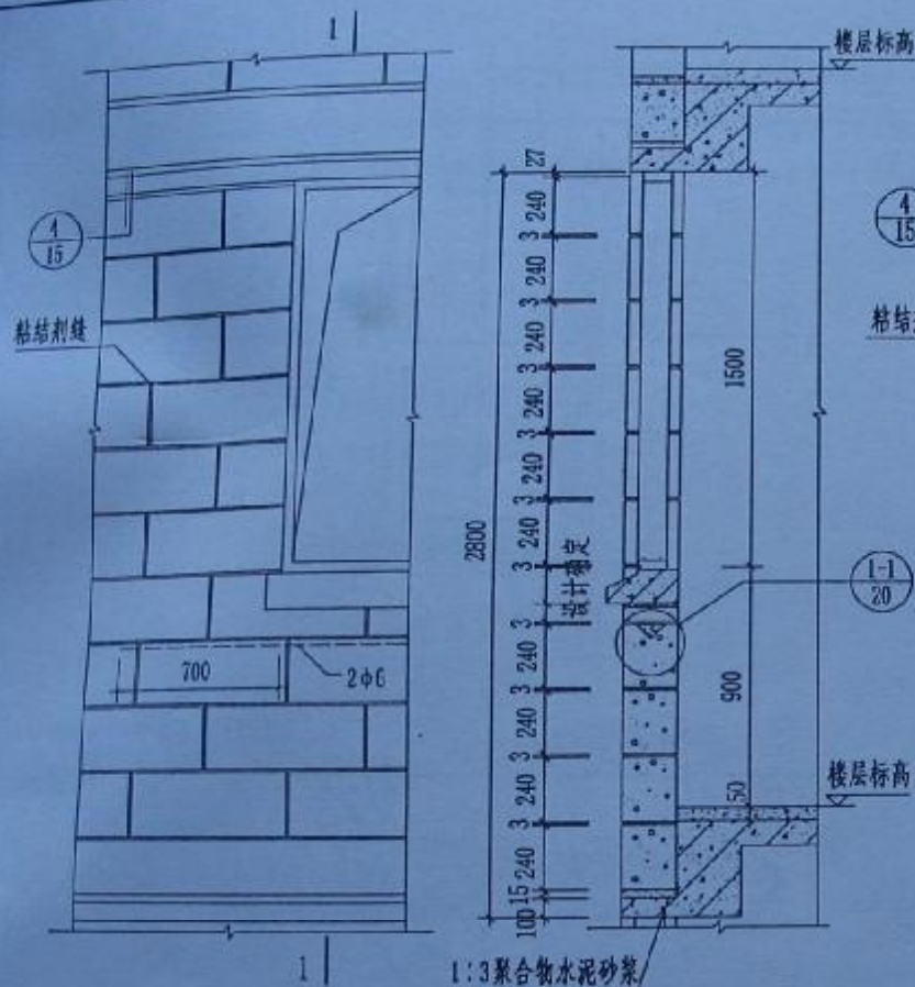
砌筑立面排块示意图 C
