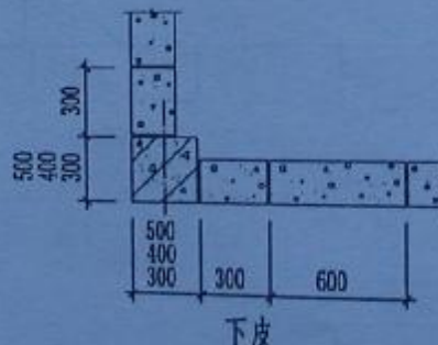
下皮(窗台线以下)
