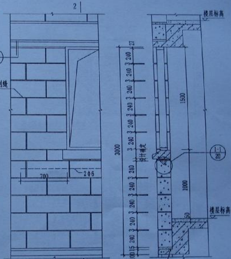
2-2 剖面
