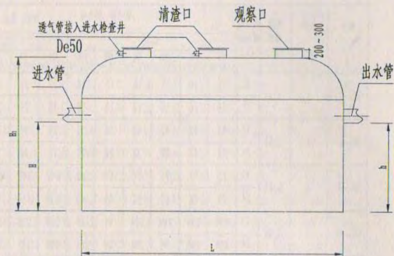
示意立面图
