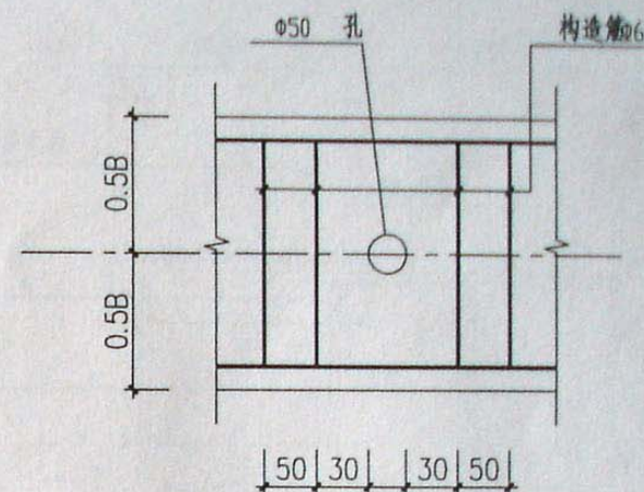
吊孔
