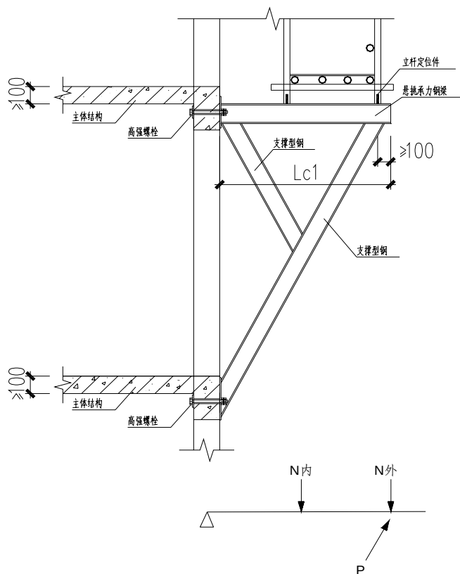
图 3.2.6 悬挑斜撑钢梁承力架构造
