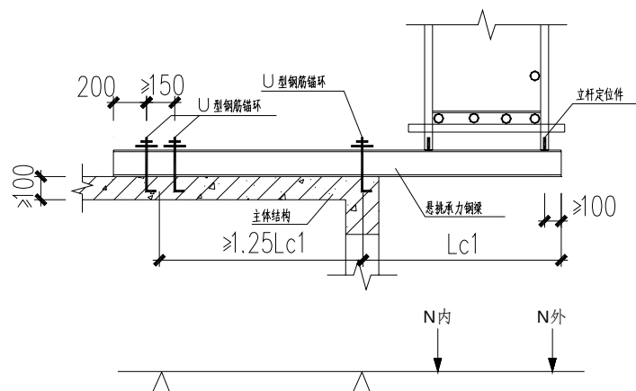
图 3.2.3 悬挑承力钢梁构造
