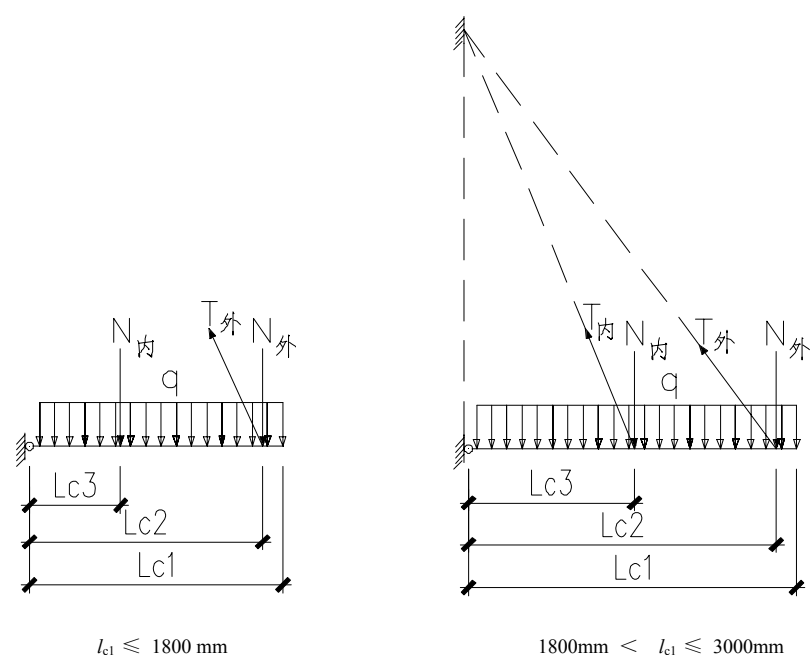
图 5.2.11 底部承力架为钢筋拉杆吊拉悬挑承力钢梁的计算示意图
