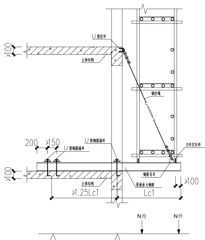
图 3.2.4 钢丝绳辅助吊拉悬挑承力钢梁构造
