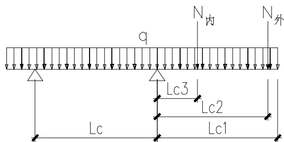
图 5.2.10 底部承力架为悬挑承力钢梁或钢丝绳辅助吊拉钢梁的计算示意图
