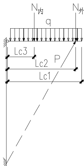
图 5.2.12 底部承力架为下撑式悬挑承力钢梁的计算示意图
