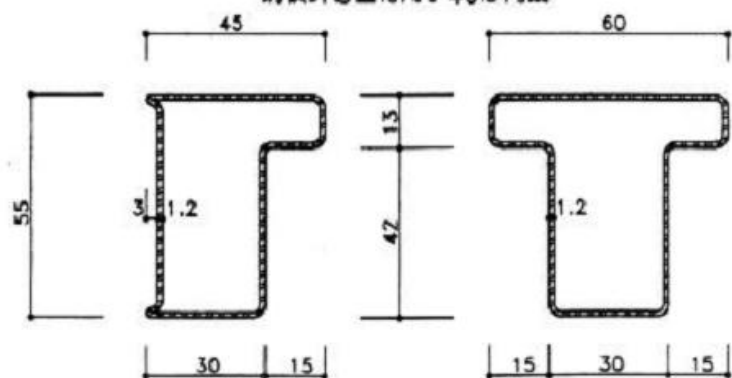
钢板折弯型材用于40厚门扇
