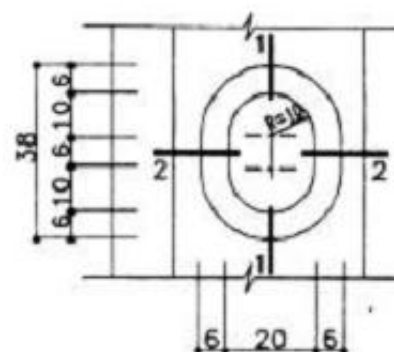
锁舌孔立面
