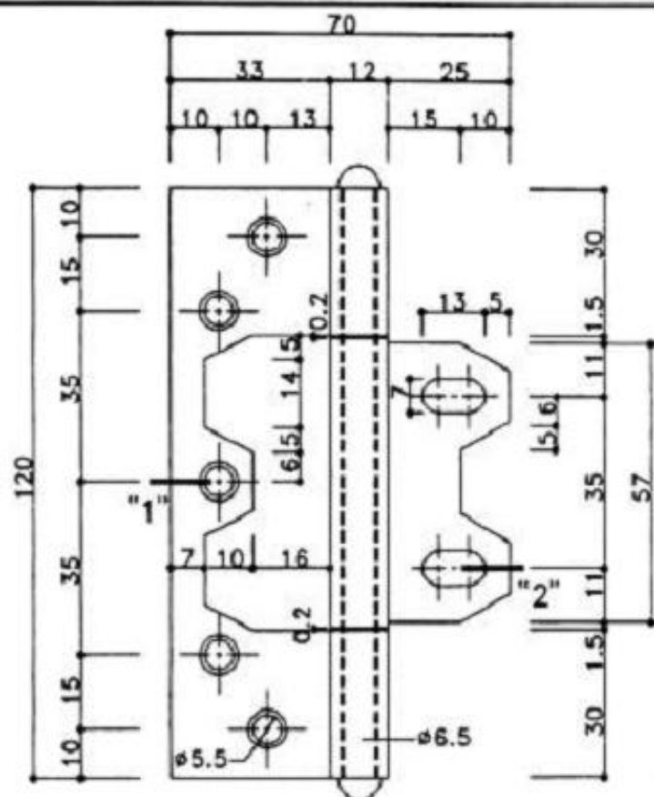
III 型铰链
