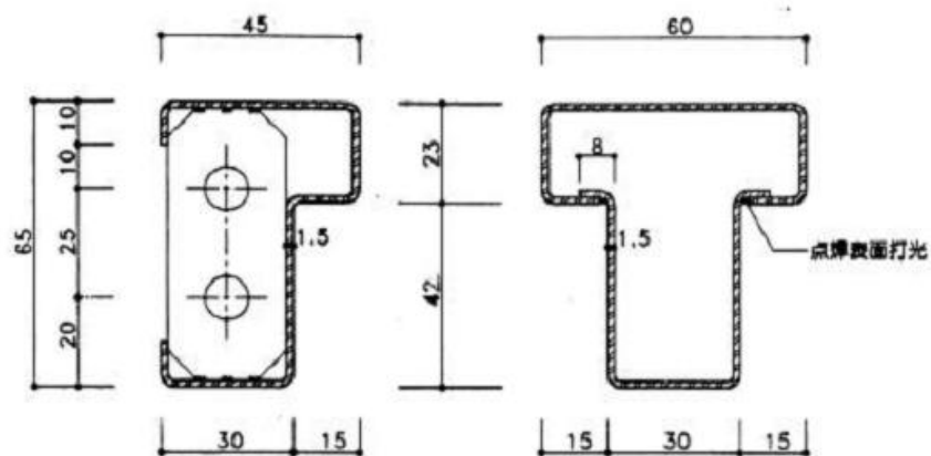
钢板折弯型材用于40厚门扇
