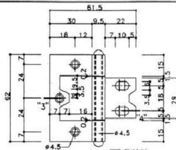
IV 型铰链
