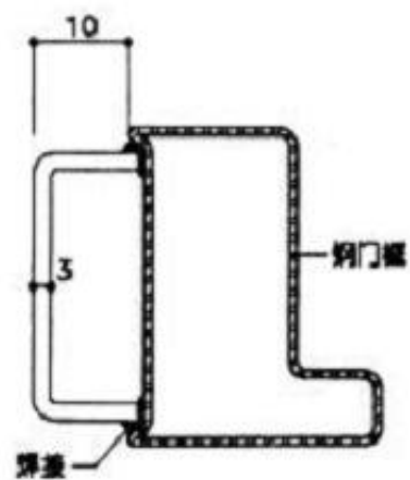
铁脚焊接位置图
