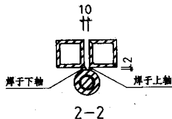
② 相联门轴
