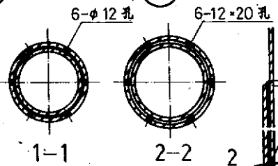
相同口径钢管对接
