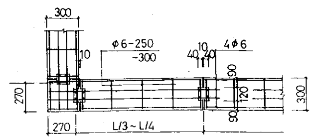
预制砼压顶板
