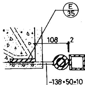
1-1 用于角钢或组合角钢边框门
