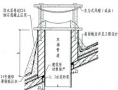
1-1 (坡屋面)
