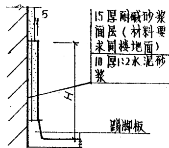
⑧ 耐碱砂浆墙裙
