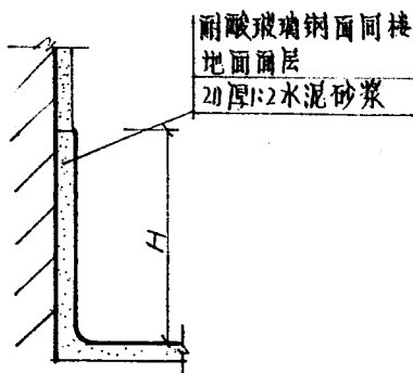
⑦ 耐酸玻璃钢墙裙
