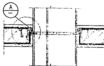
② 烟气道承托做法
