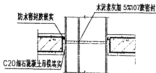
① 烟气道端口做法
