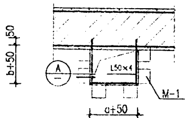
⑥ 烟气道承托角钢平面布置 (二)
