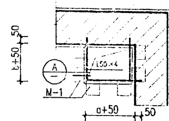
⑤ 烟气道承托角钢平面布置 (一)
