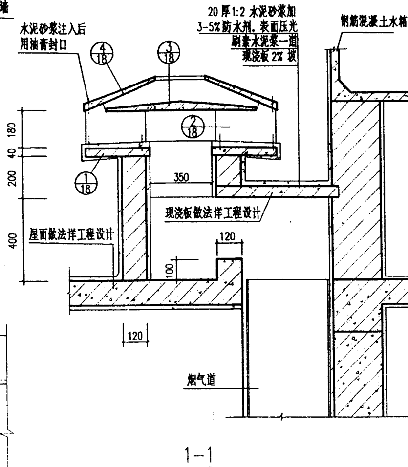
风帽与屋顶水箱交接处节点详图
