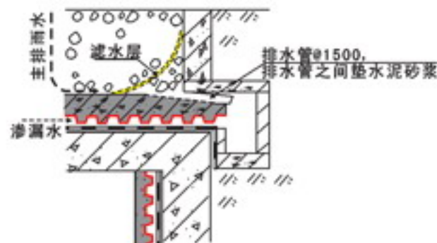
⑧ 顶板整体采用(构造B)
