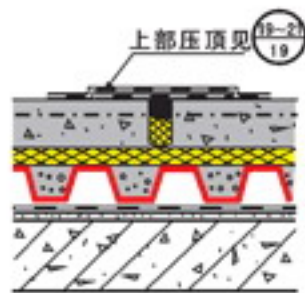
③② 倒置保温分仓缝
