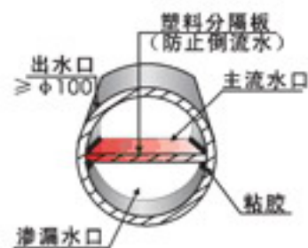
A~A出水口
