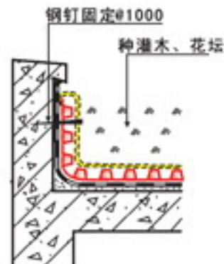
③ 女儿墙(一)
