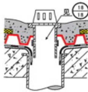
③4 倒置保温垂直落口
