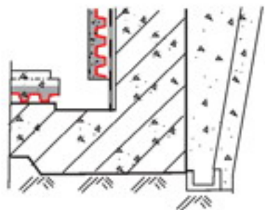
⑯ 底板与内墙排水转角
