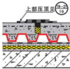
②8 正置保温分仓缝
