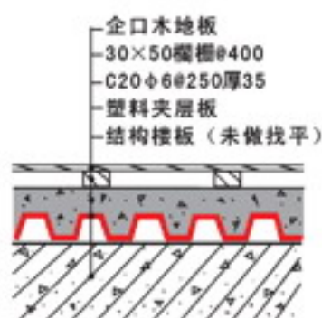
③⑬ 架空地坪上 铺栅木地板 (可以避免结构楼板钻孔洞)
