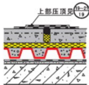
③2 倒置保温分仓缝
