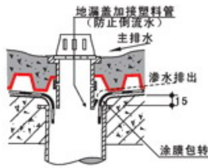
⑱ 双层垂直落水口
