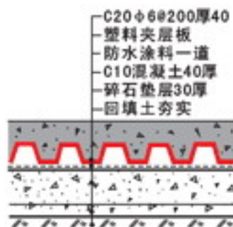
③⑯ 底层防潮地坪
