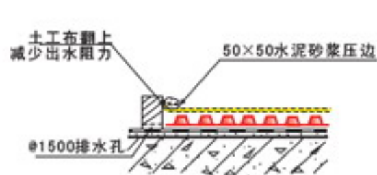
⑫ 端部收口
