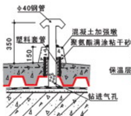
②4 透气管
