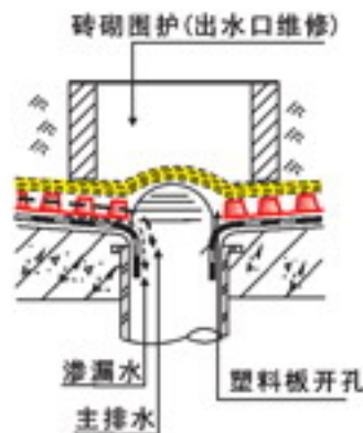
⑥ 垂直出水口(一)
