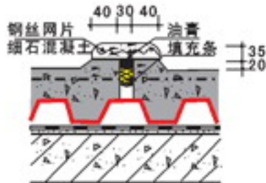
②1 分仓缝 (做法三)
