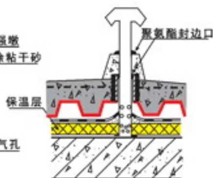
②5 加保温层透气管
