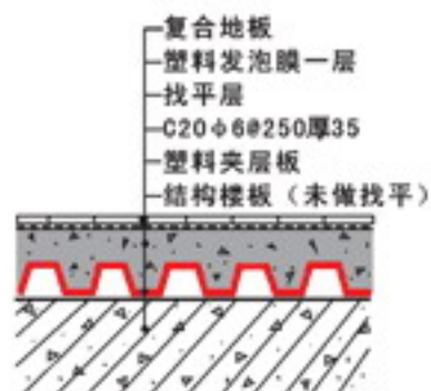
③⑪ 架空地坪上 铺复合板
