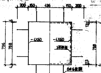
边框平面 (右面表示竖切型)
