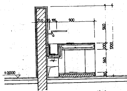
2-2 (单面)
