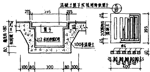
室内排水沟剖面
