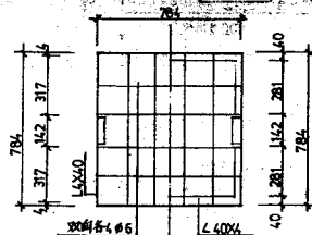
盖板钢筋骨架平面布置 (右面表示竖切型)
