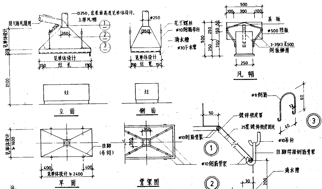
厨房排气罩 (一)
