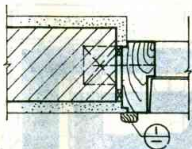
120砖墙固定门框
