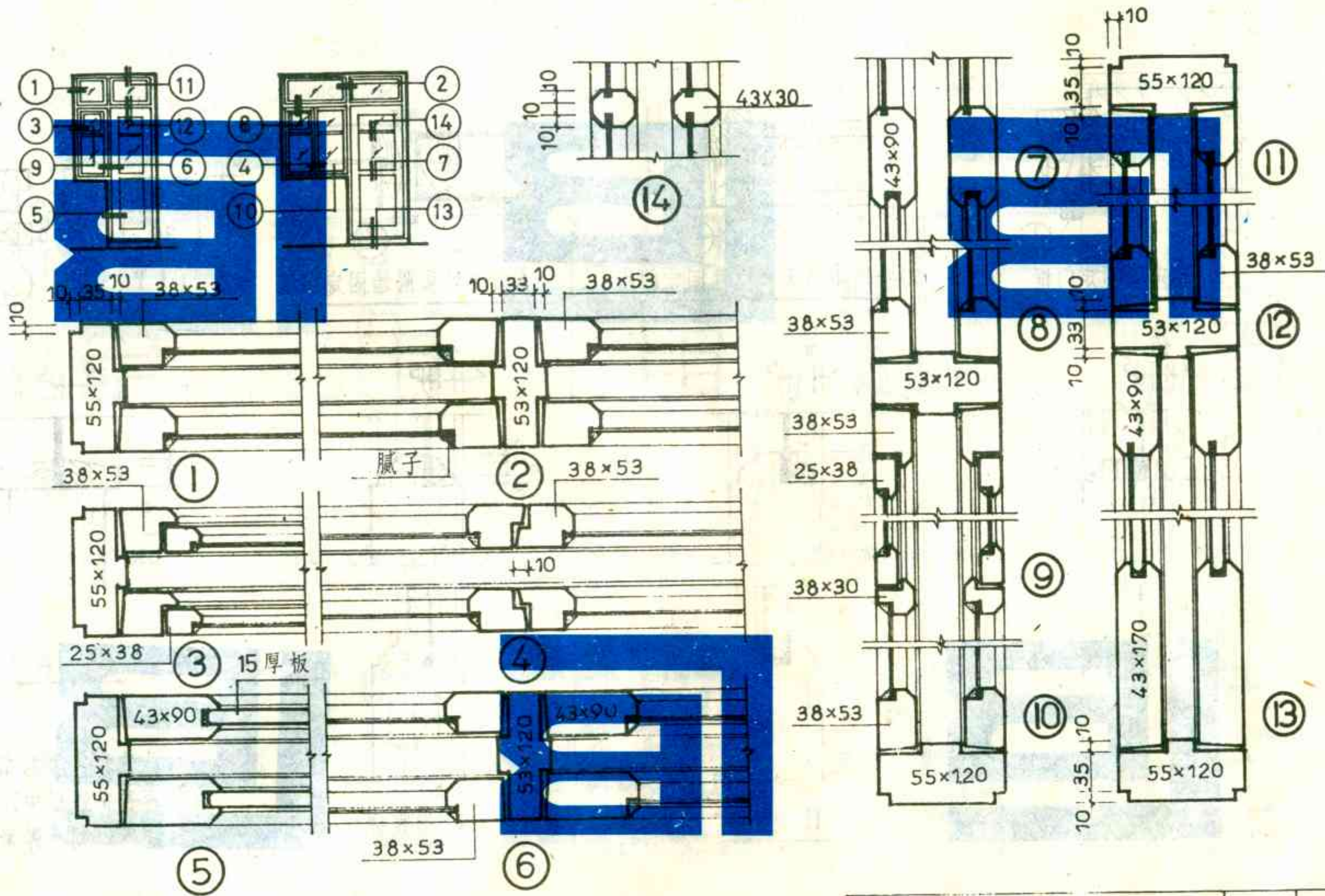
M6 双层阳台门节点详图
