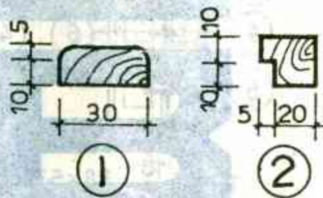
木骨架轻质隔墙固定门框
