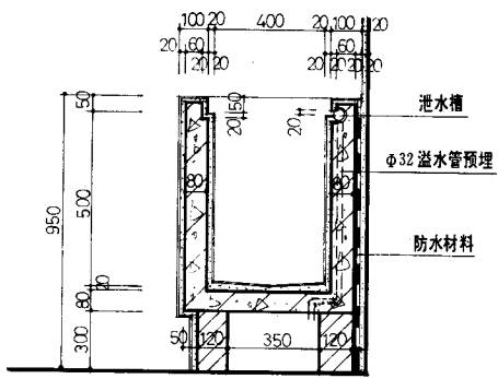
1—1 剖面
