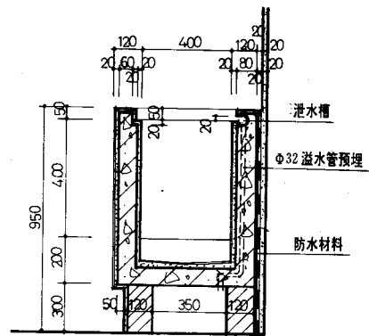
2—2 剖面
