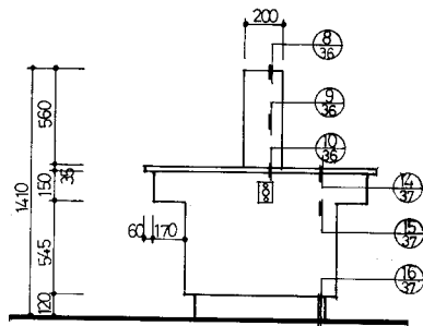
侧立面
