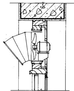
轴流风机安装示意
