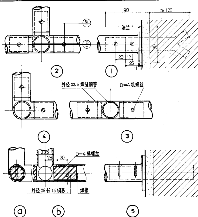
吊杆大样
