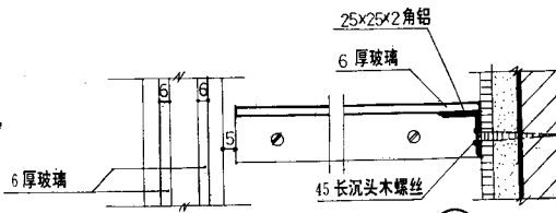
1—1 剖面
