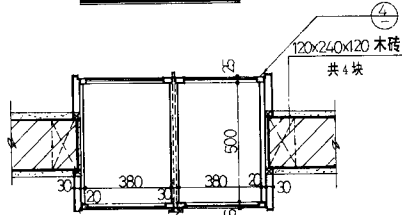
传片箱立面
