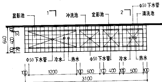
洗片池平面
