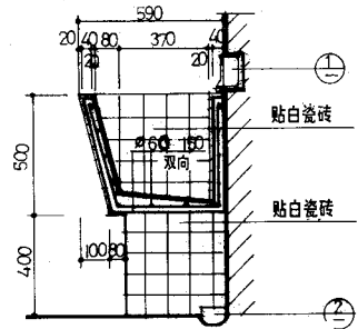
1—1 剖面
