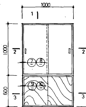
1—1 器械柜立面
