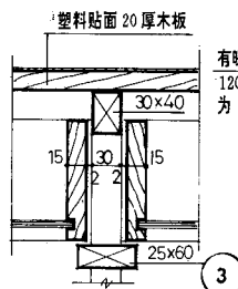
挂号、收费窗口大样
