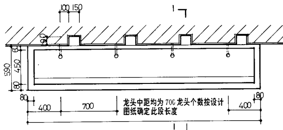
洗手池平面
