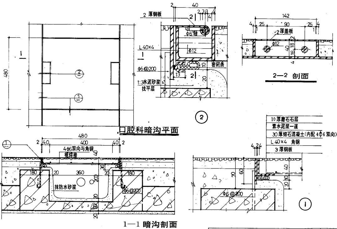
口腔科暗沟及检查盖
