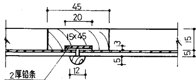
A—A 剖面
