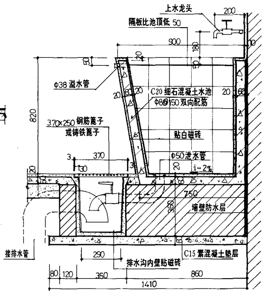
1—1 剖面
