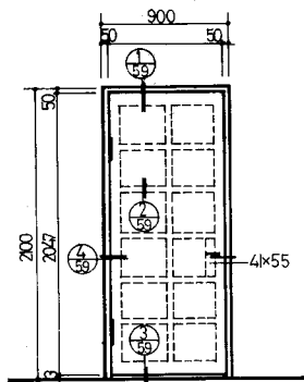
门立面
