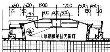
1-1 观察台剖面
