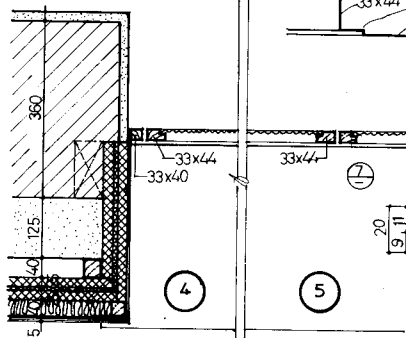
隔电窗立面
