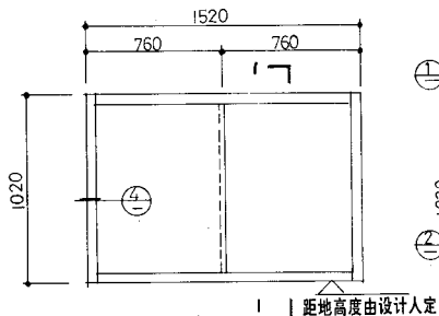
器械柜立面
