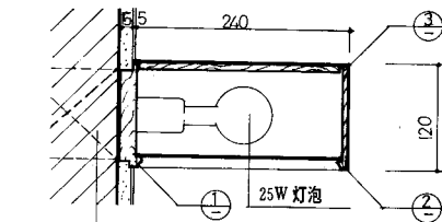
1—1 剖面
