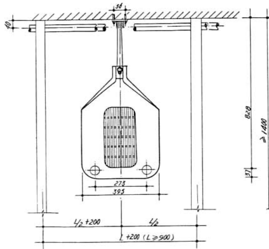
平面分隔图
