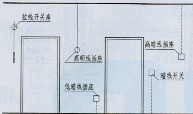
电器开关、插座位置示例
