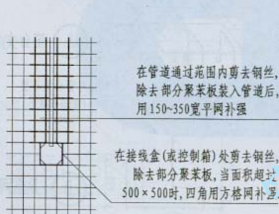
③ 预埋管线做法
