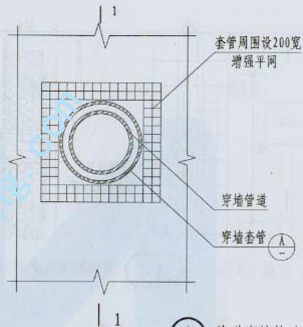
① 管道穿墙构造
