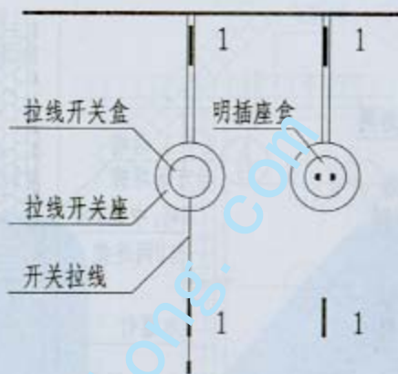
① 明线拉线开关、插座
