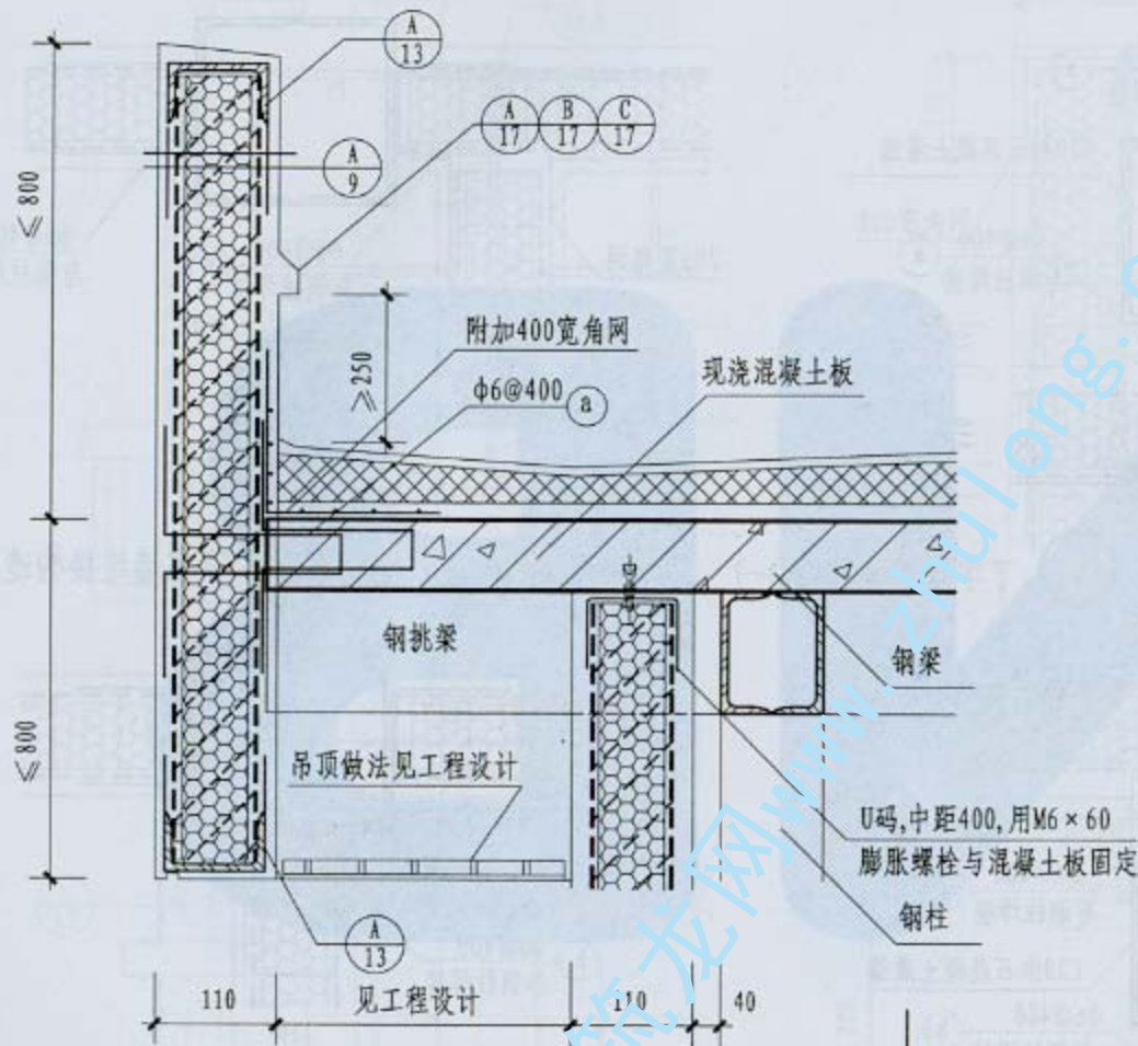
1 挑檐檐墙构造
