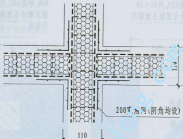
② 板墙与板墙十字连接构造
