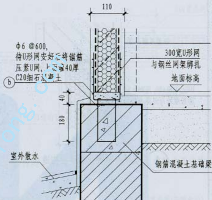
3 板墙与基础连接构造(三)
