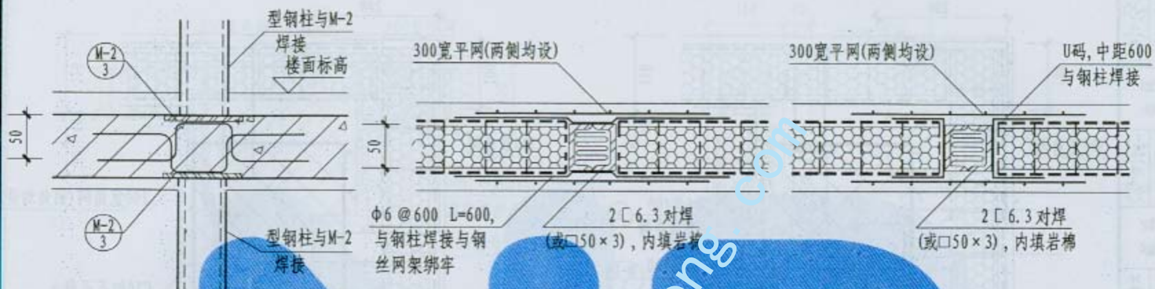
① 加劲柱与楼板(梁)连接构造
