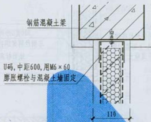
① 板墙与混凝土梁连接构造(一)
