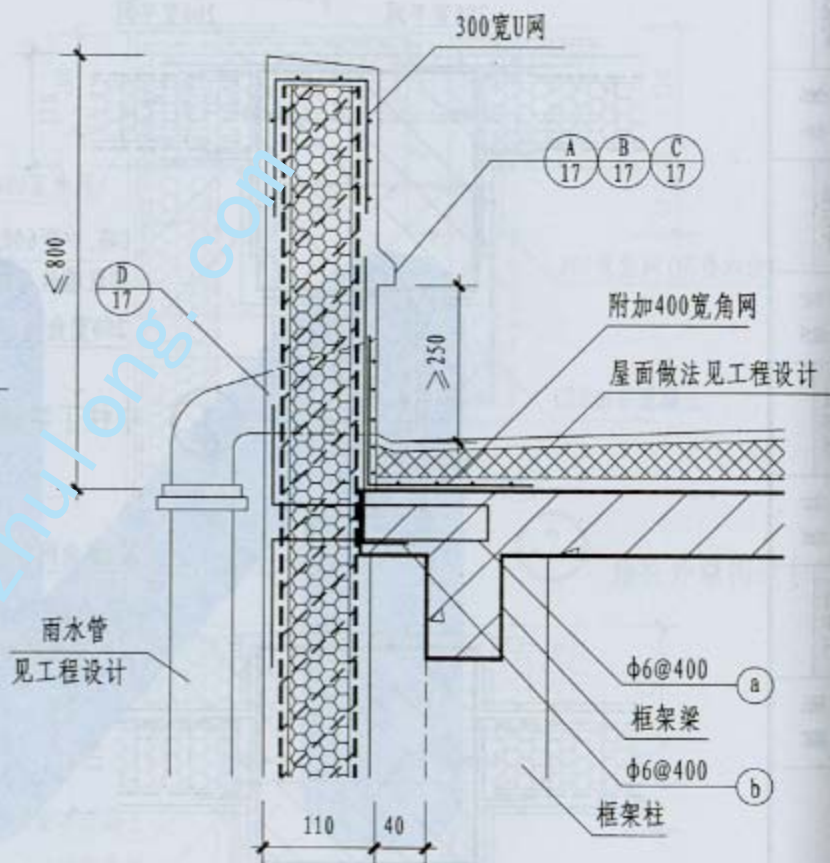
2 女儿墙构造(二)
