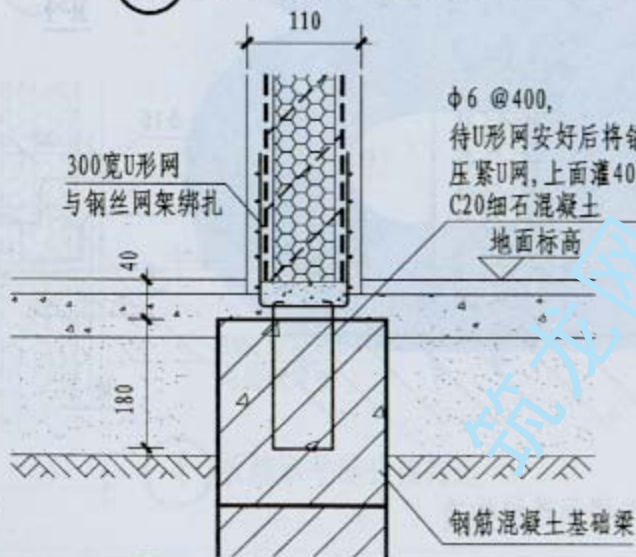
2 板墙与基础连接构造(二)
