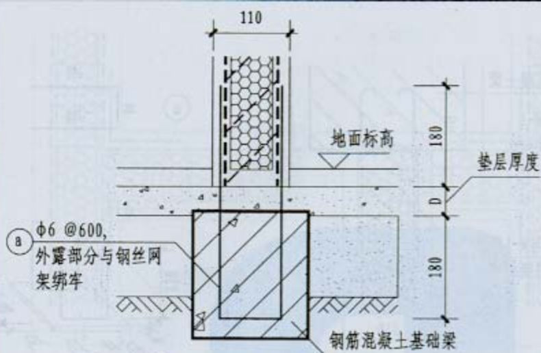
1 板墙与基础连接构造(一)
