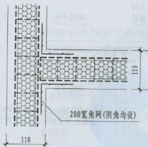
① 板墙与板墙丁字连接构造
