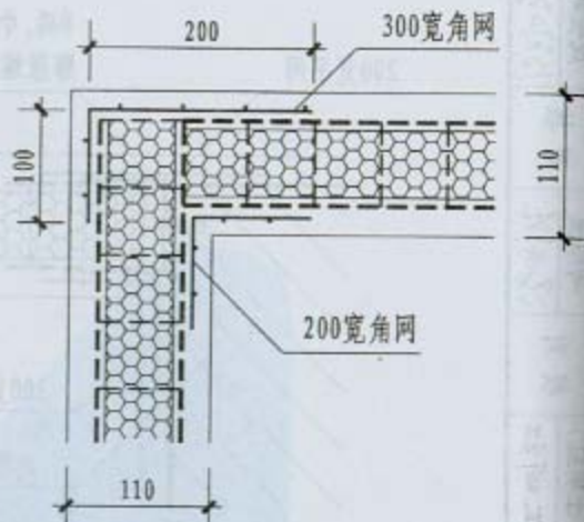
③ 板墙与板墙转角连接构造
