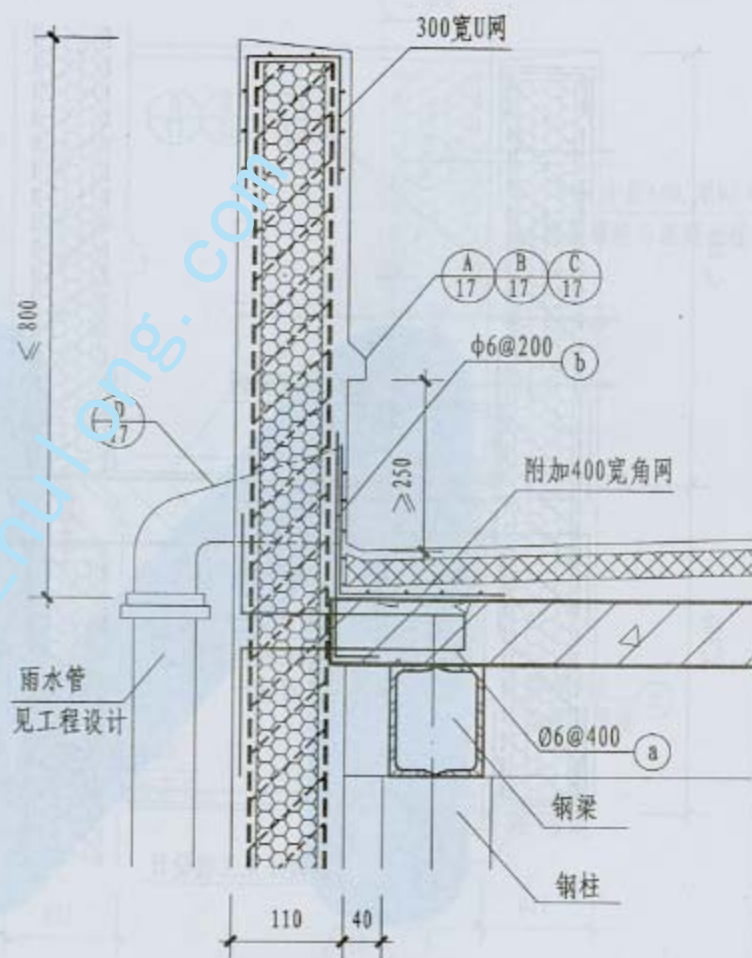
2 女儿墙连接构造(钢筋混凝土屋面)
