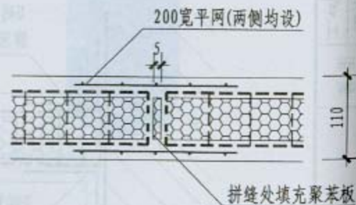
⑥ 外墙板竖缝拼接构造
