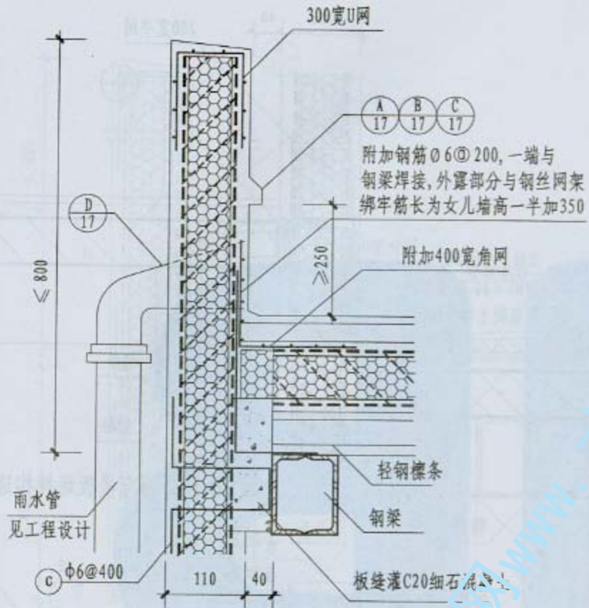
1 女儿墙连接构造(钢结构屋面)
