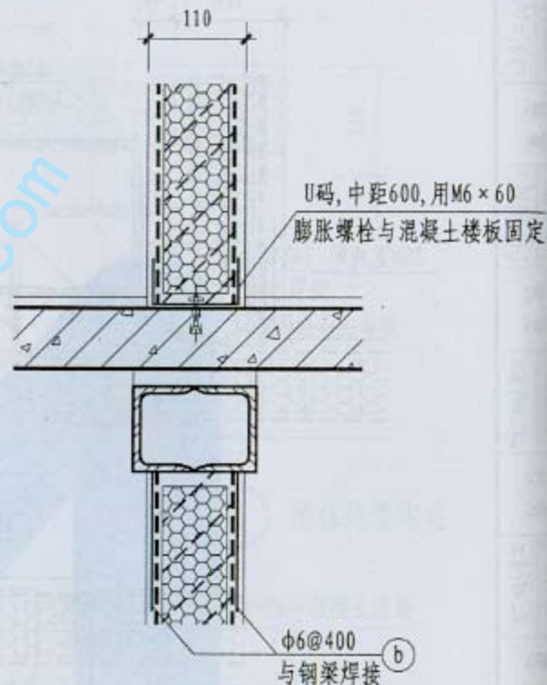
2 楼板连接构造
