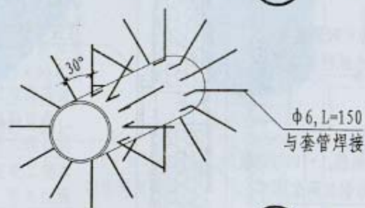
② 穿墙套管
