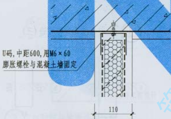
③ 板墙与顶板连接构造
