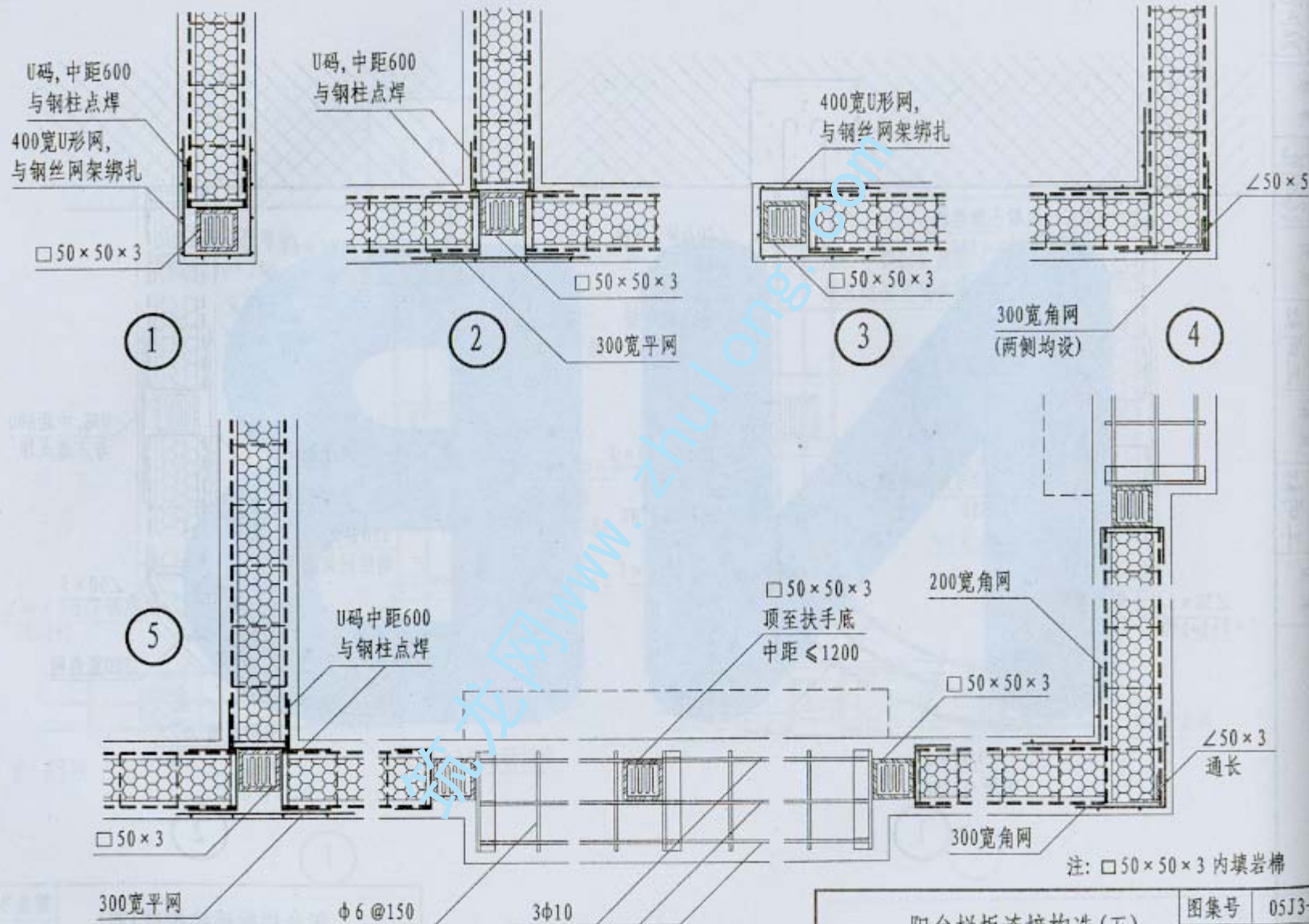
阳台栏板连接构造(五)
