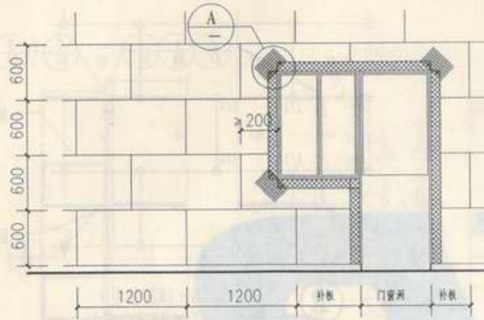
板材门窗洞口排板示意
