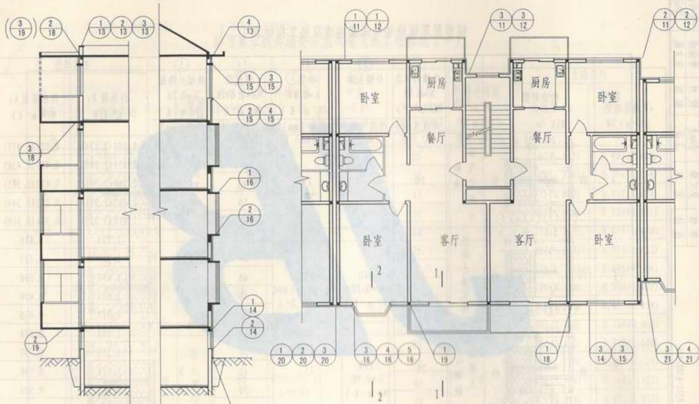
外保温墙体平面索引
