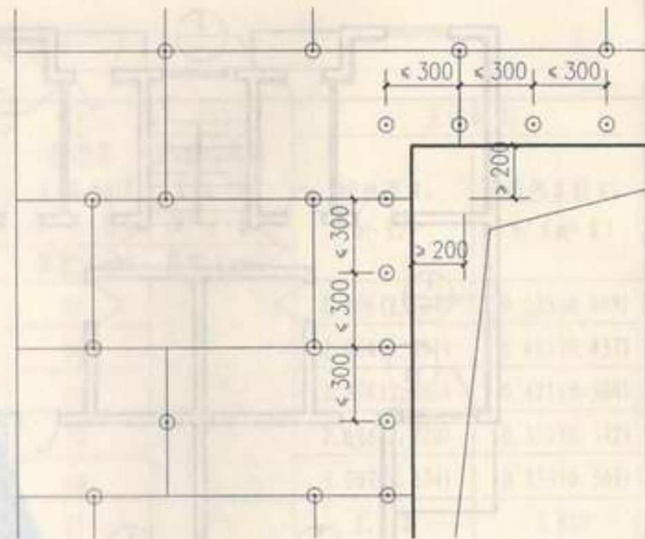
1 洞口及边角固定件布置图
