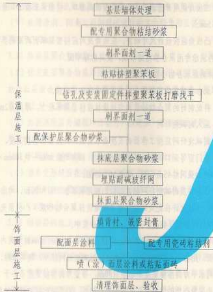
图2.2-1 施工工序流程图
