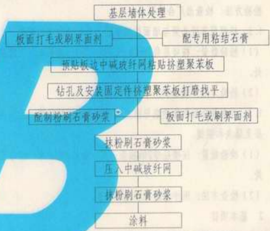
图2.2-1 施工工序流程图
