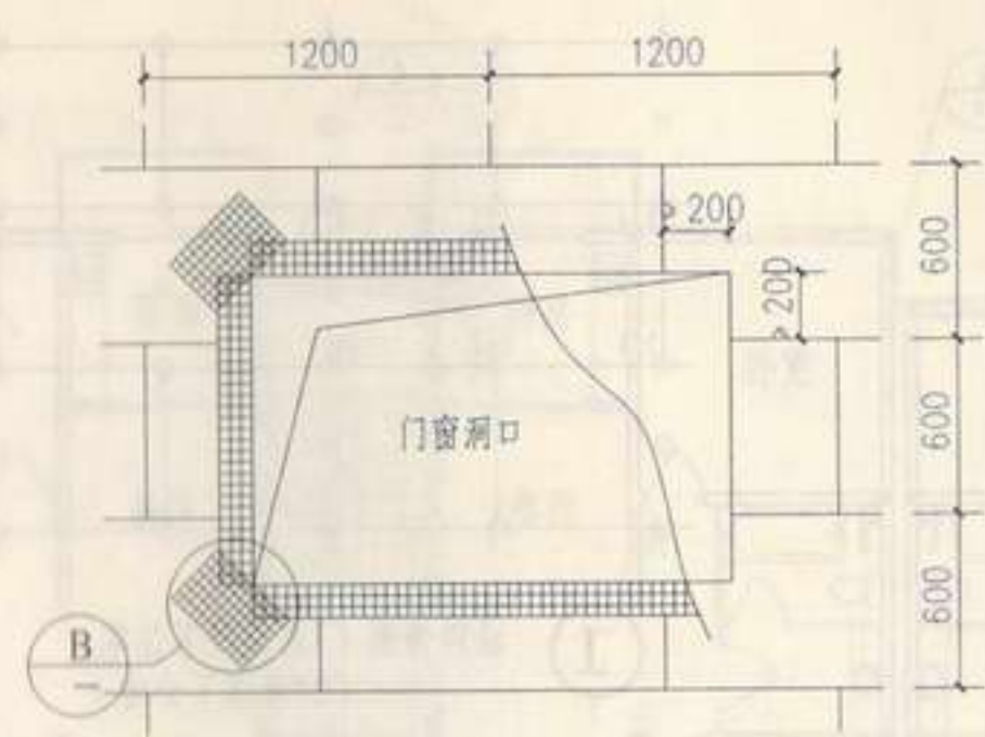
门窗洞口耐碱玻纤网加强示意
