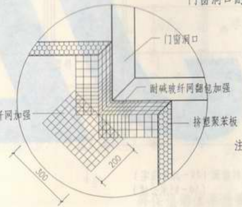
门窗洞口耐碱玻纤网加强示意
