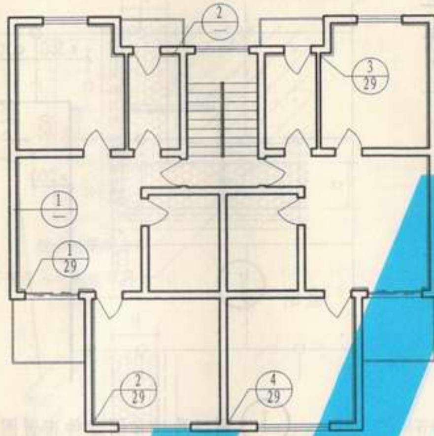
内保温墙体平面索引
