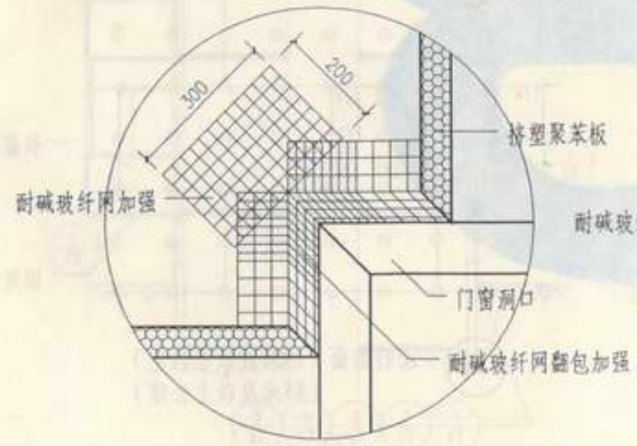
板材门窗洞口排板示意
