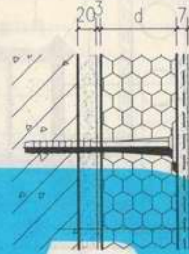
① 内保温墙体构造 (涂料饰面)
