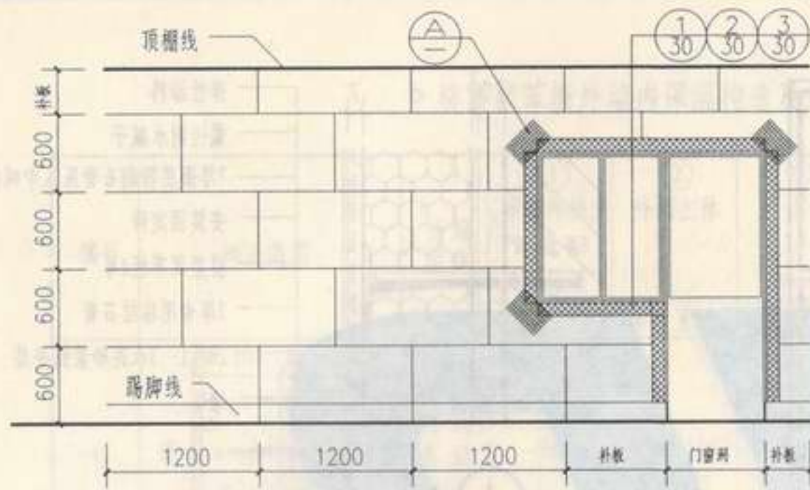
门窗洞口挤塑聚苯板排板
