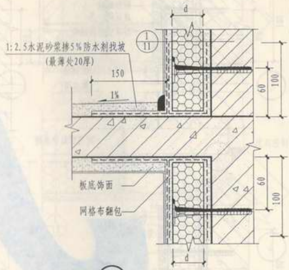
③ 阳台楼面(空调机搁板)
