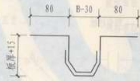
A 金属盖缝板
