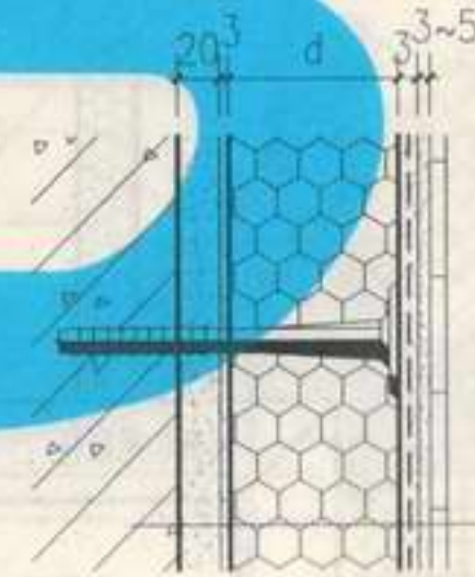
② 内保温墙体构造 (面砖饰面)
