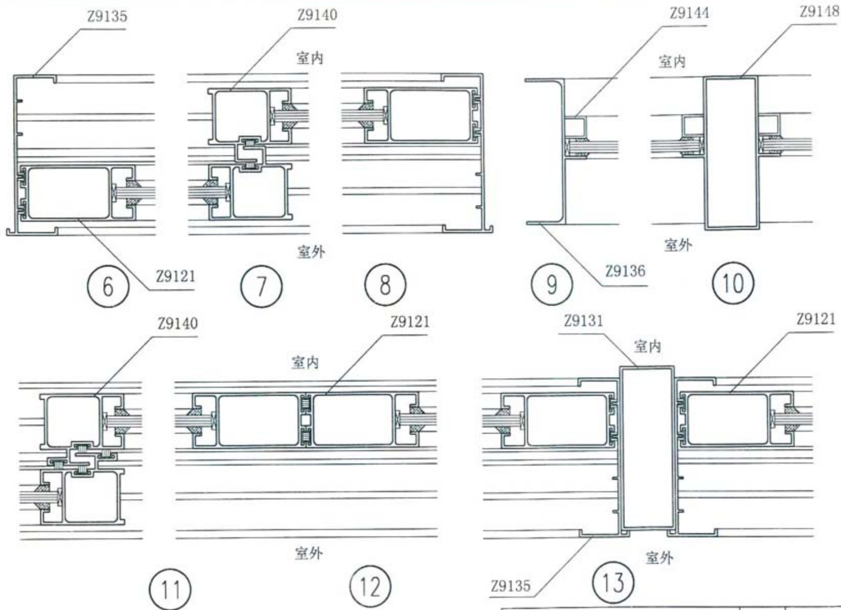
不带纱无框窗节点详图(二)
