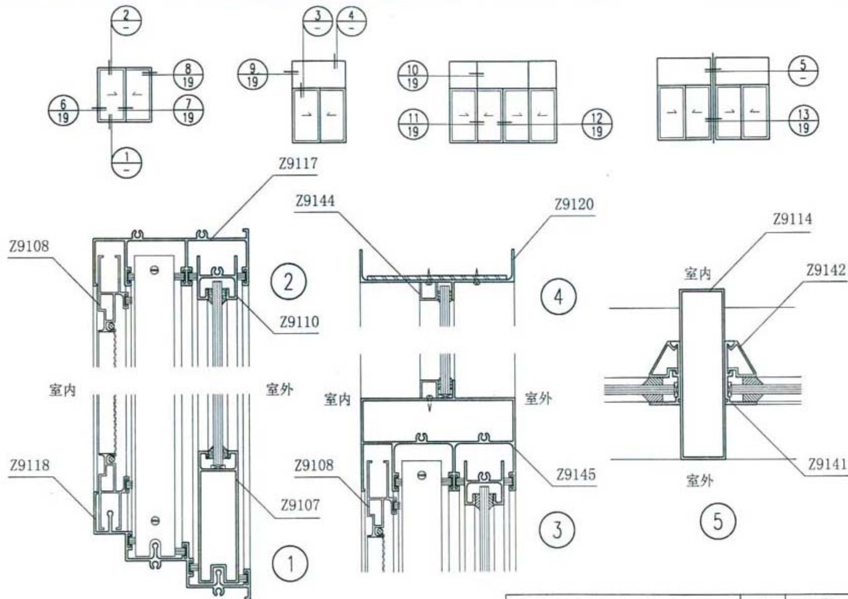
带纱无框窗节点详图 (一)
