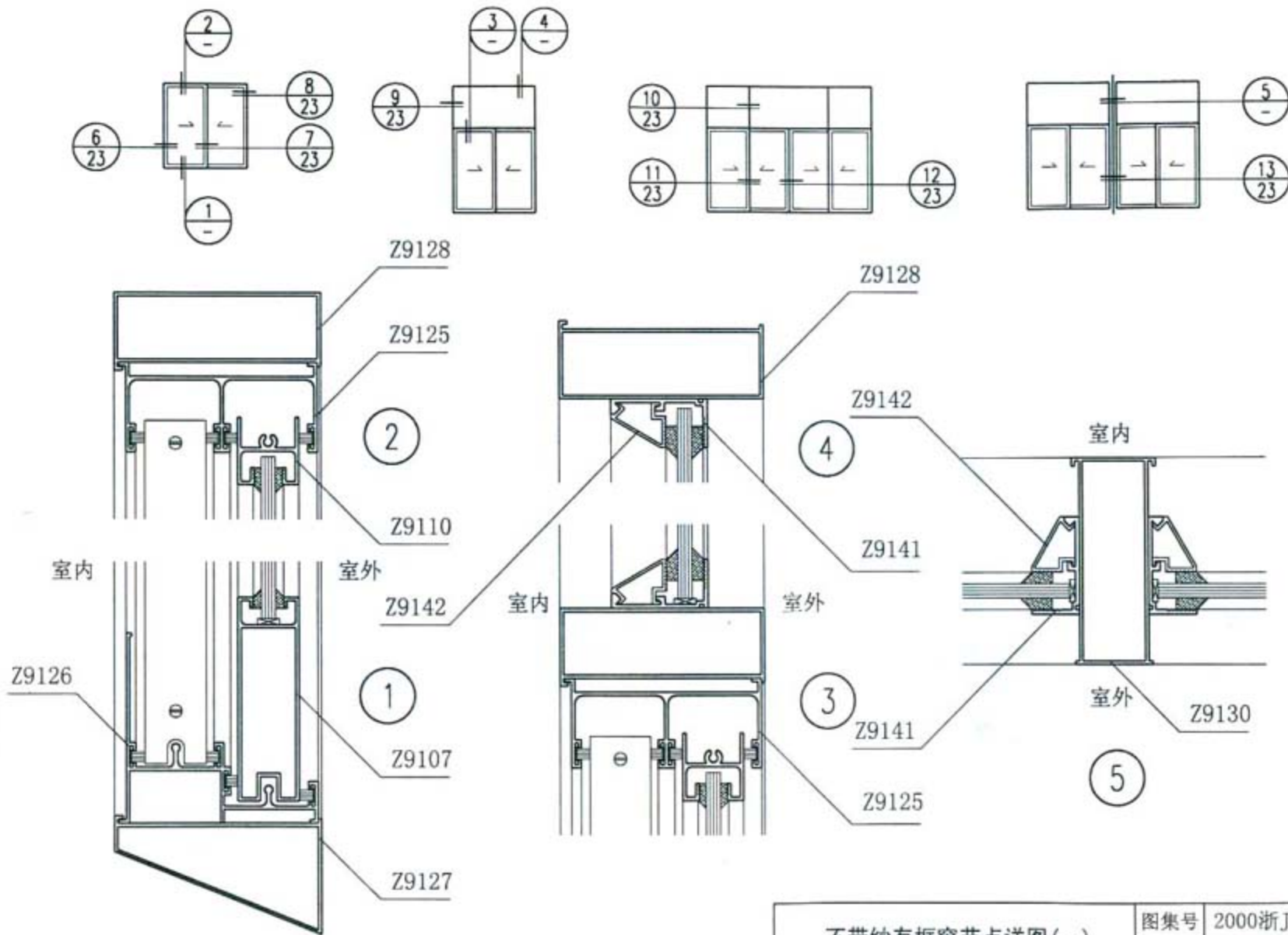
不带纱有框窗节点详图(一)
