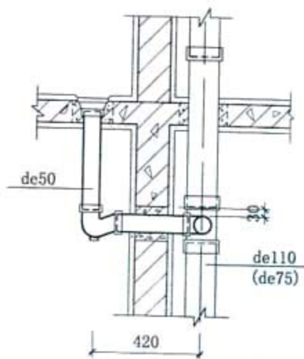
① 立面
