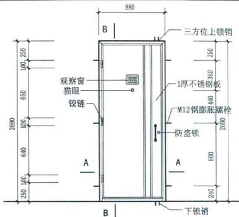
钢质防盗门(不锈钢)立面
