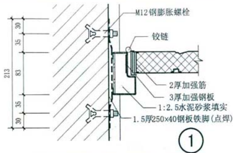
门框与墙侧居中安装(门向室内开启)
