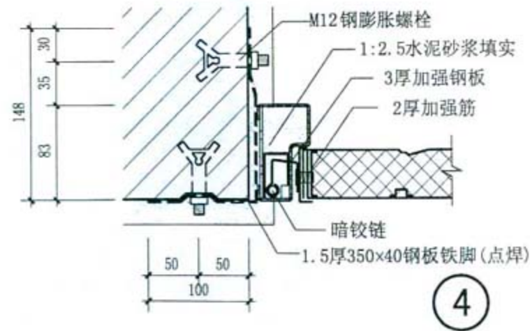
门框与墙外侧齐平安装(门向室外开启)
