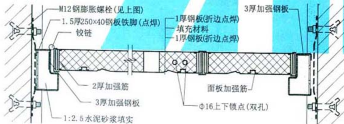
A-A 剖面
