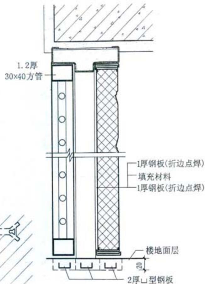
B-B 剖面
