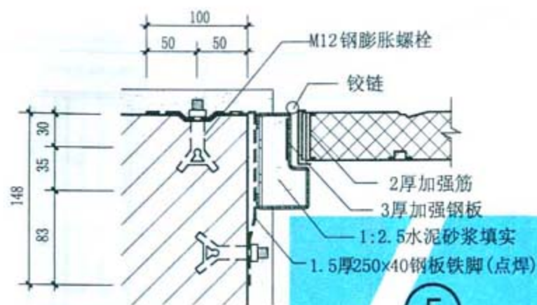
门框与墙内侧齐平安装(门向室内开启)
