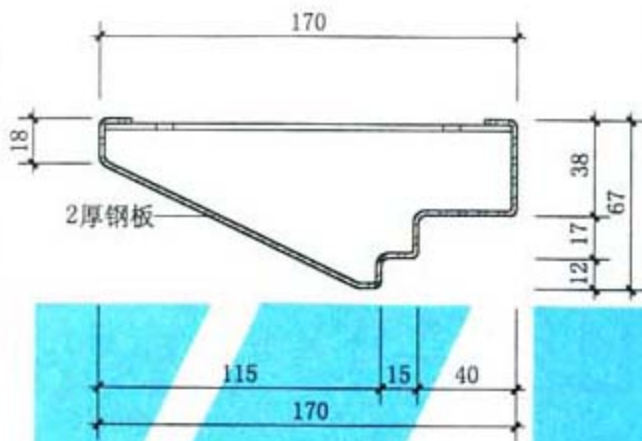
III型门框断面
