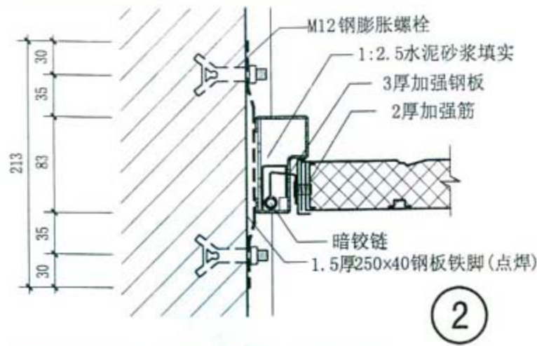
门框与墙侧居中安装(门向室外开启)
