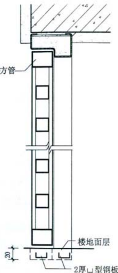
B-B 剖面
