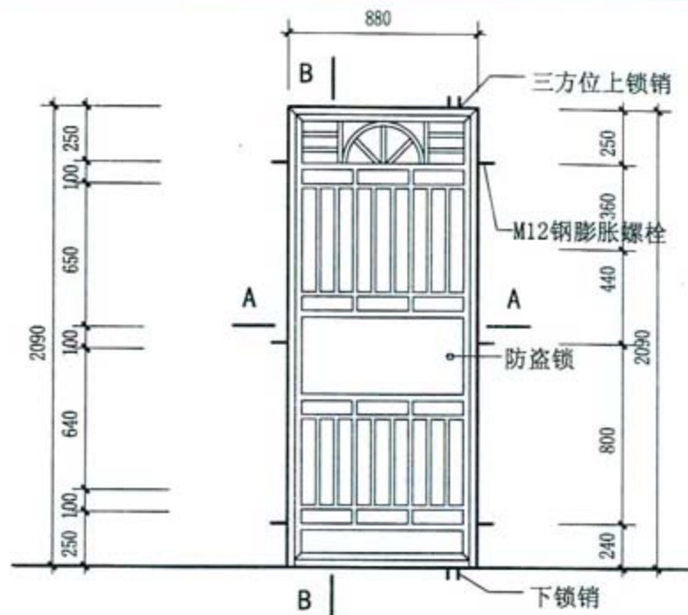
栅栏防盗门立面
