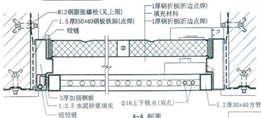
复合防盗门(一框二门)详图
