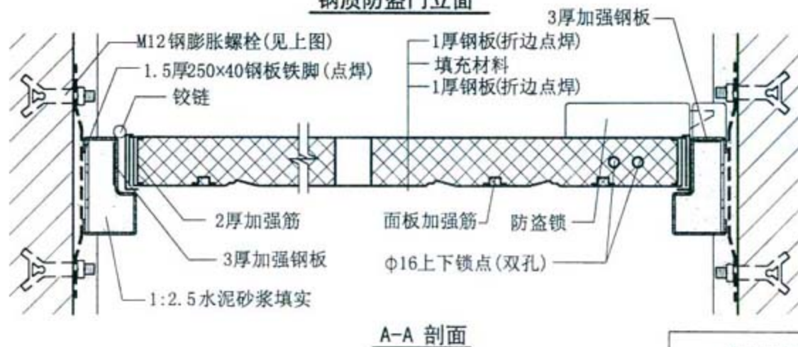
钢质防盗门详图(一)
