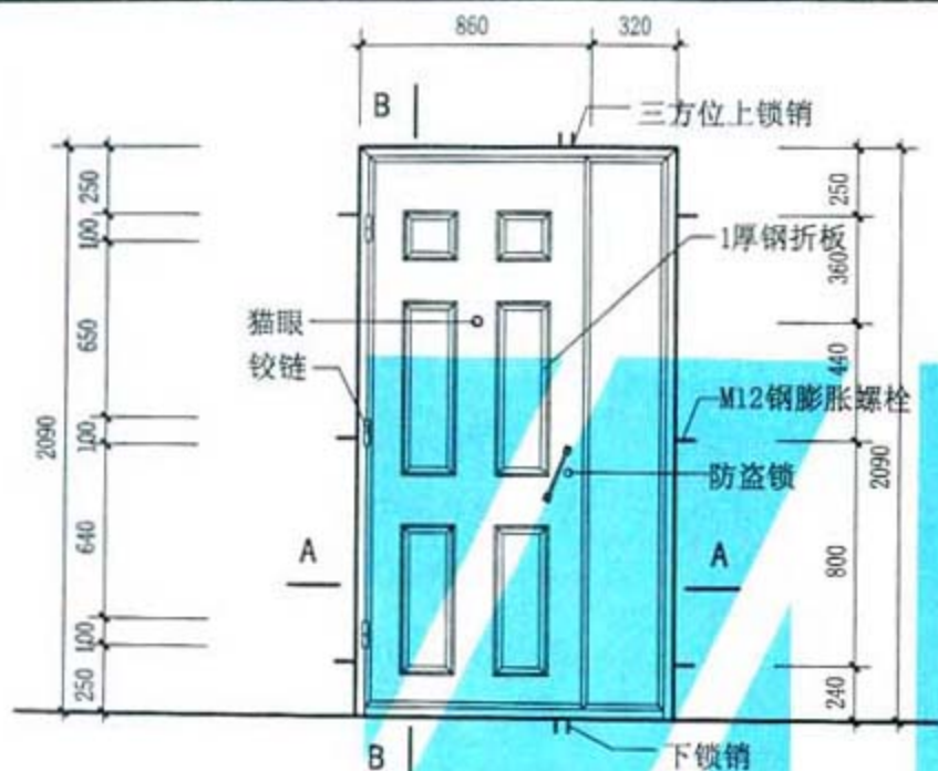
钢质防盗门立面
