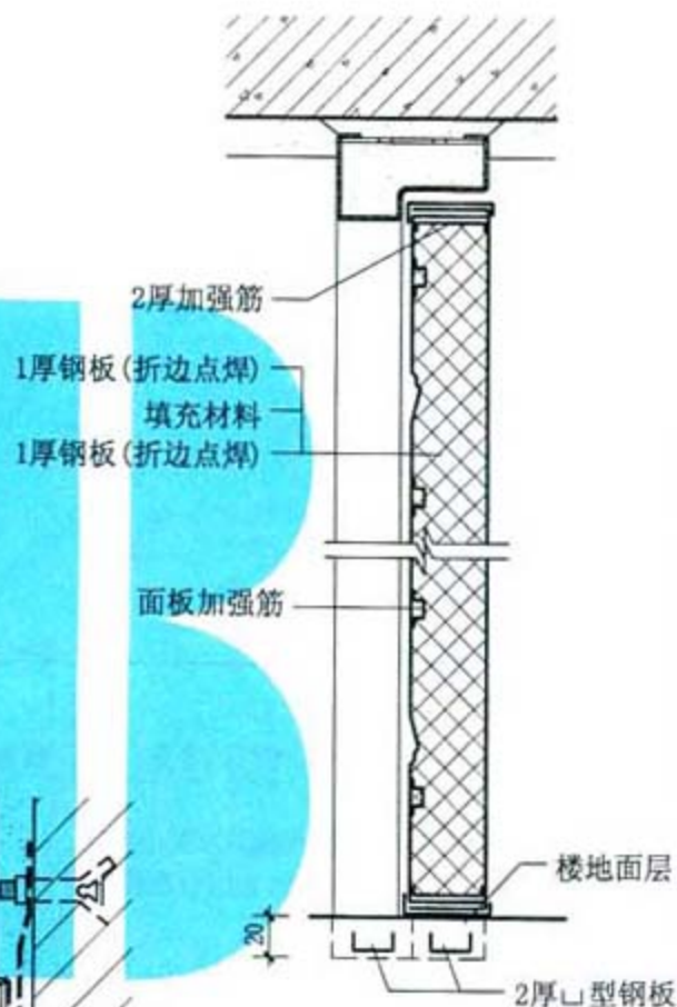
B-B 剖面
