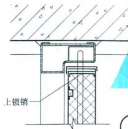
门框顶部安装节点
