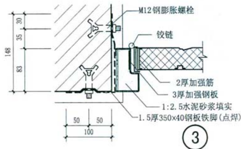
门框与墙外侧齐平安装(门向室内开启)
