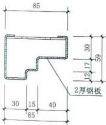
II 型门框断面
