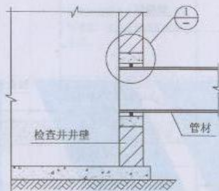
管道与检查井井壁连接(二)
