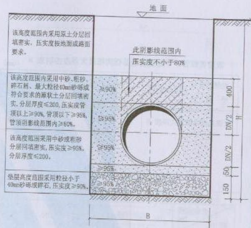
管道基础及回填土要求(二)
