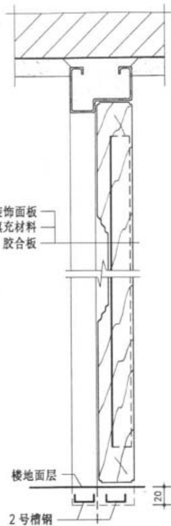
B-B 剖面
