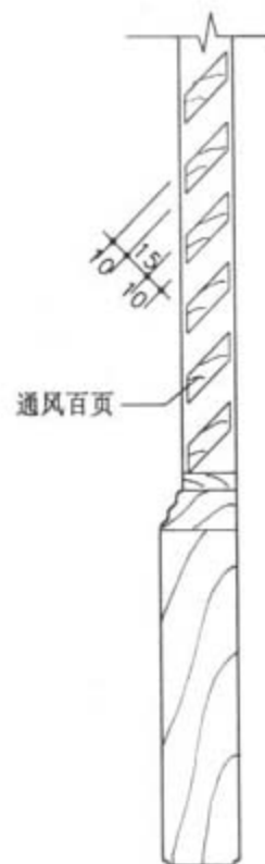
卫生间门立面(二)
