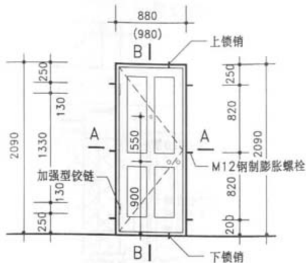
钢木防盗门立面
