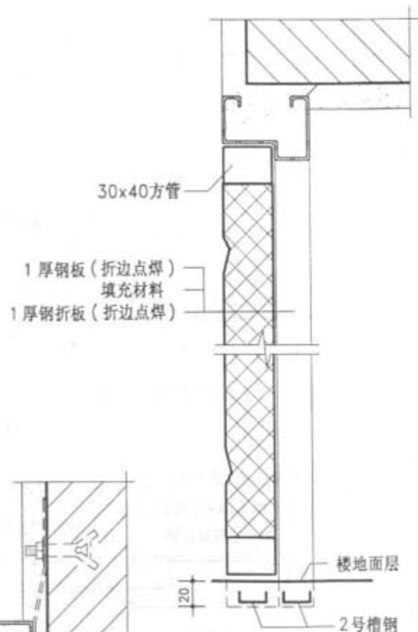
B-B 剖面
