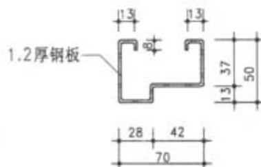
门框料
