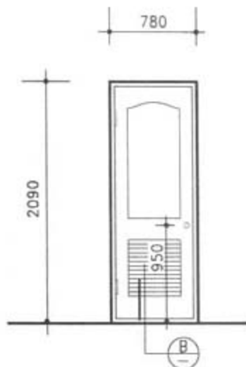
卫生间门立面(一)
