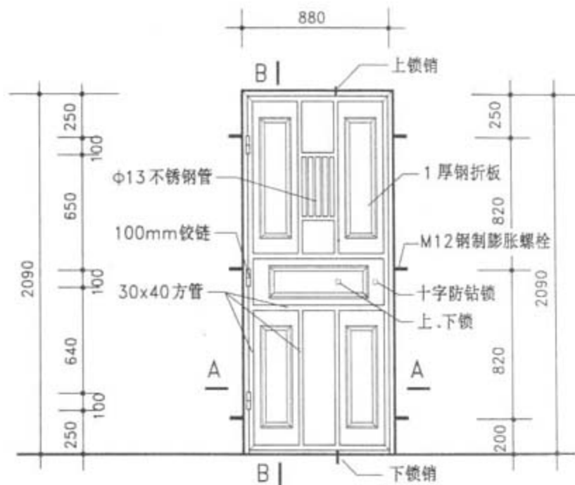
全封闭防盗门立面
