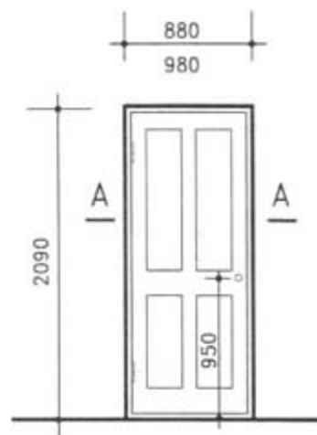
装饰内门立面
