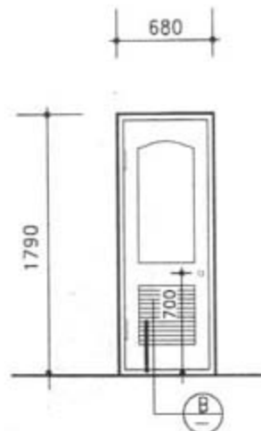
卫生间门立面(二)
