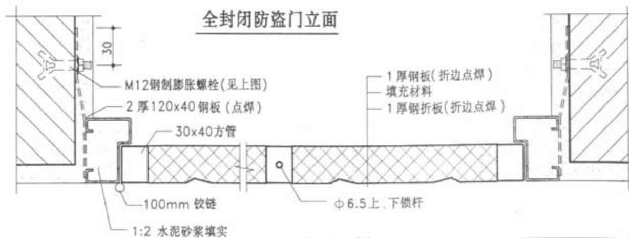
A-A 剖面
