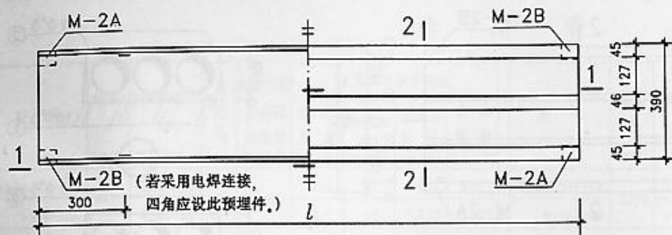
YRKB 4-XX-XXX 二孔板平、剖面
