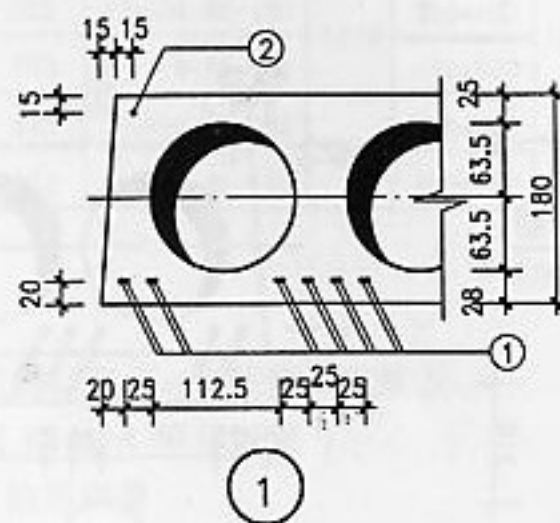
二孔板详图
